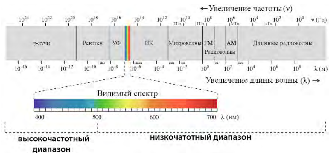
Рисунок 2. Электромагнитный спектр
