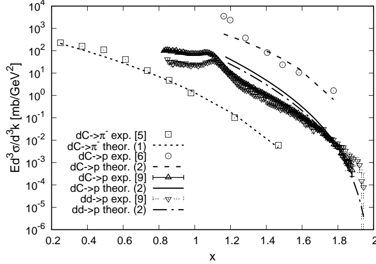
Рис. 3. Сравнение результатов теоретических расчетов инклюзивных сечений по формулам (1) и (2) (кривые) с экспериментальными данными (точки) по рождению отрицательно заряженных пионов и протонов при фрагментации дейтрона в реакциях d+d и d+C из работ [5, 6, 9, 10] (см. пояснения в тексте).
