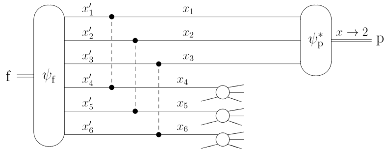
Рис. 2. Образование кумулятивных протонов за счет механизма когерентной коалесценции трех кварков флуктона [15–17].
