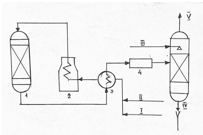
Рис 2.-Технологическая схема регенерации катализатора гидроочистки паровоздушной смесью.
