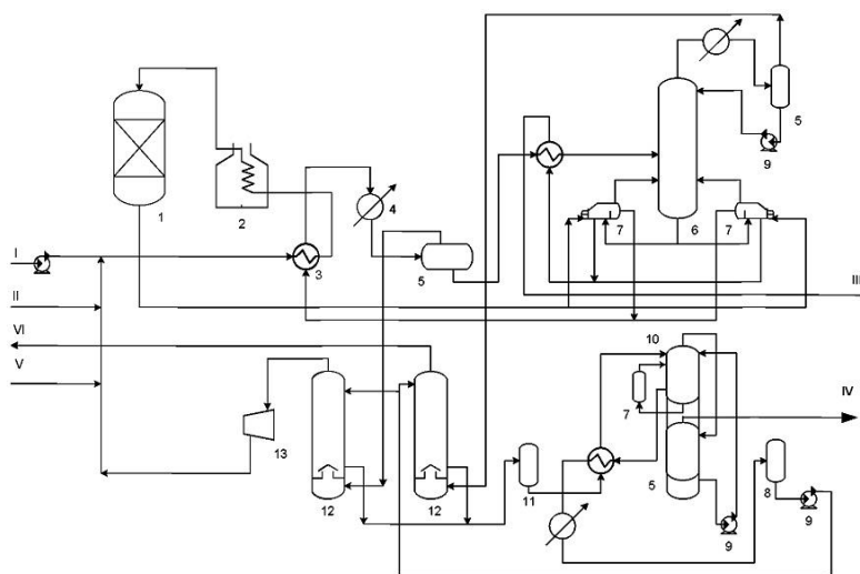
Рис 1. - Технологическая схема регенерации катализатора гидроочистки классическим способом:
