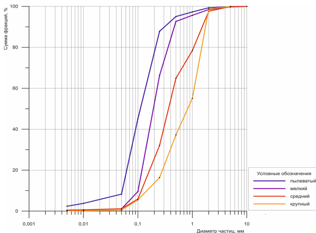
Рисунок 4 – Интегральная кривая гранулометрического состава песков нерасчищенного комплекса палеогеновых отложений (Р) области влияния ОАО «Гомельский химический завод»
