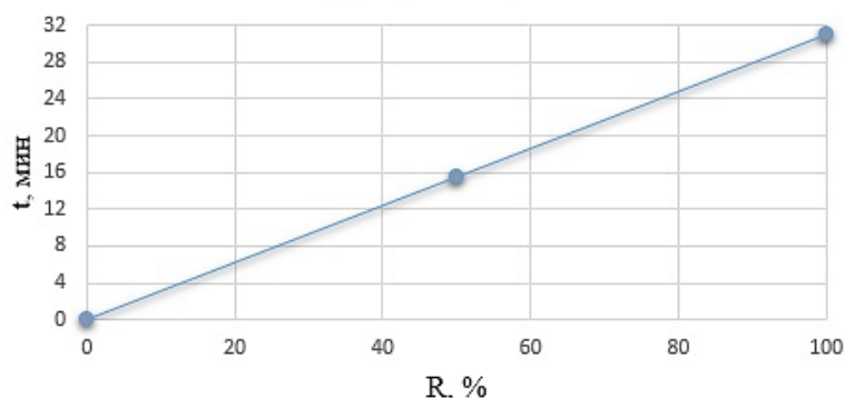
График кинетики размокания грунта №4 (фосфогипс)
