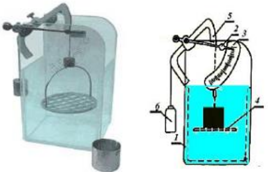
1 – корпус; 2 – стрелка; 3 – шкала; 4 – сетка; 5 – рычаг; 6 - противовес
