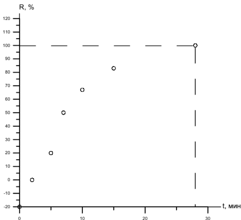
Рисунок 3 – Кинетика размокания глинистого грунта
