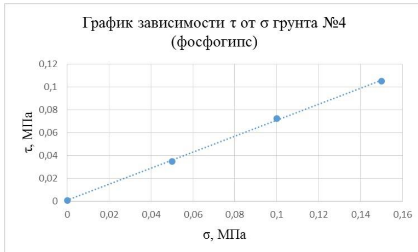
Рисунок 2 – График зависимости \tau от \sigma фосфогипса
