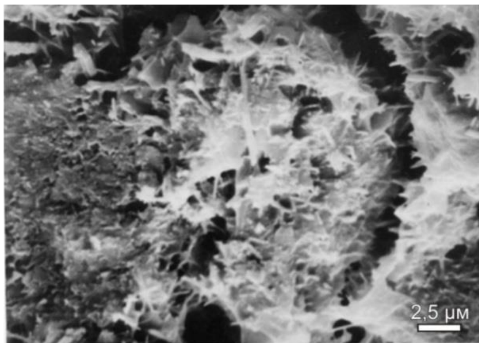
Рисунок 1 – Формирование кристаллических новообразований и микродефектов в поровом пространстве зологрунта. 28 суток твердения (фото В.Н. Соколова)
