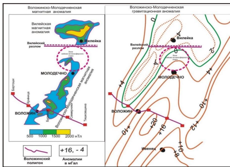
Рисунок 2 – Схема Лидского полигона, секущего вкрест простирания Воложинско-Молодечненскую аномалию. Аномальное гравитационное и магнитное поля - по материалам 1980 – 1984 гг.
