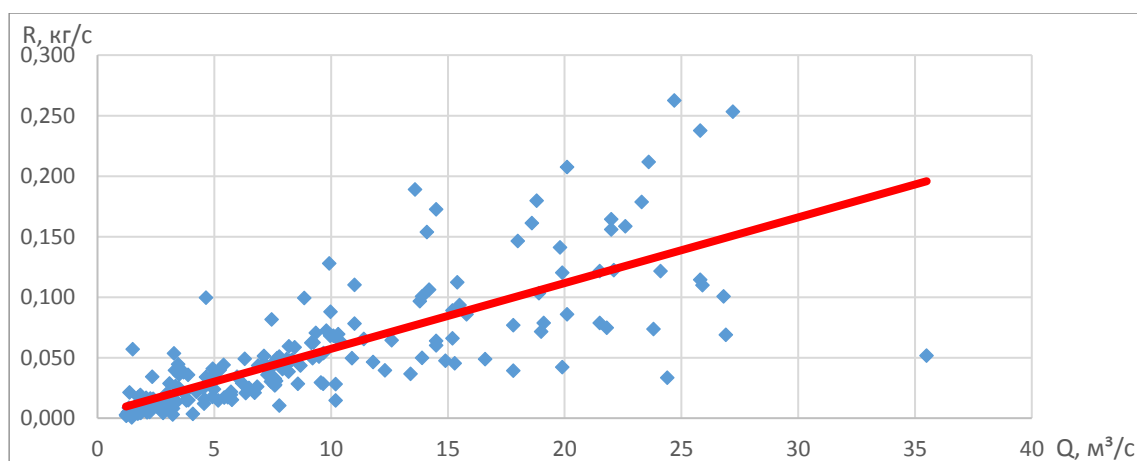
Рисунок 2 – График связи среднегодовых расходов воды ( Q \text{ м}^3/\text{с} ) и наносов ( R \text{ кг/с} ) объединенного ряда значений
