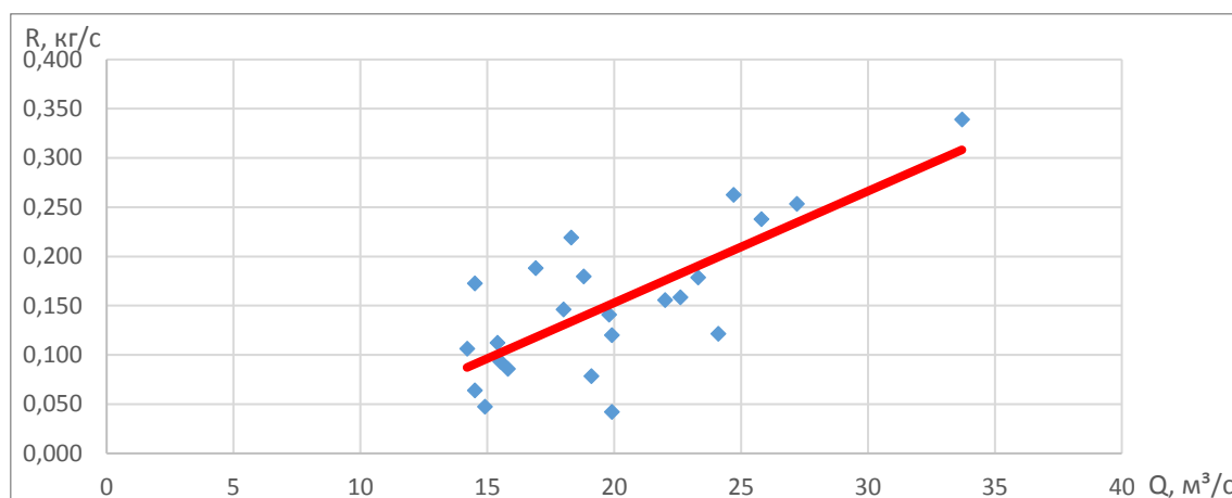
Рисунок 1 – График связи среднегодовых расходов воды ( Q м 3 /с) и наносов ( R кг/с) р. Виляя – г. Вилейка
