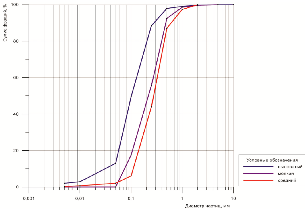
Рисунок 2 – Интегральная кривая гранулометрического состава песков среднечетвертичные моренные отложения днепроовского подгоризонта (gQ2pr1-dn) области влияния ОАО «Гомельский химический завод»
