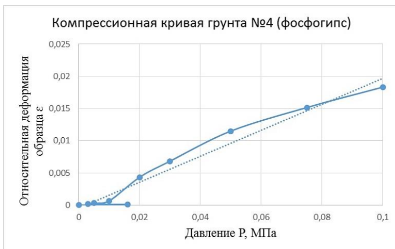
Рисунок 1 – Компрессионная кривая фосфогипса
