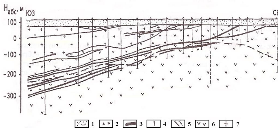
Рисунок 3- Диабазовое месторождение. Профильный поперечный разрез (составил М.Г. Левый)[1]
