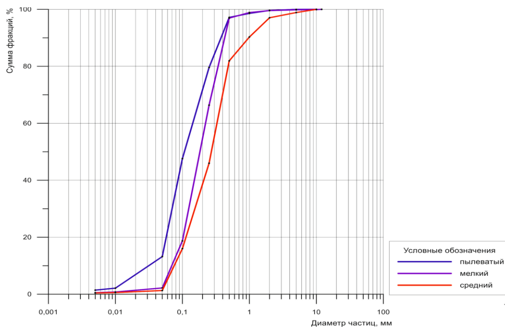
Рисунок 1 – Интегральная кривая гранулометрического состава песков нерасчлененного комплекса водноледниковых и аллювиальных отложений средне-верхнечетвертичного возраста ( f,lgQ_2pr_1-dn^s + a_2Q_3pz_3 ) области влияния ОАО «Гомельский химический завод»
