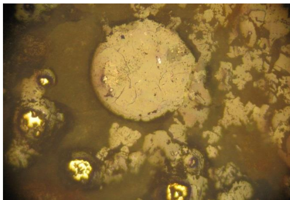
Рисунок 5 – Глобуль настурана (светло-серое в центре); желтое – пирит. Аншлиф. Скважина № 1449 – 278,0 м. Увеличение 300× Фото автора
