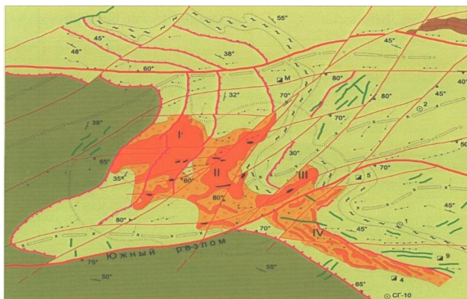
Рисунок 1 – Схематическая геологическая карта Мурунтауского рудного поля. (А.К.Воронков, Г.В.Касавченко, И.А.Образцов и др.). (Условные обозначения обозначены на рисунке 2)
