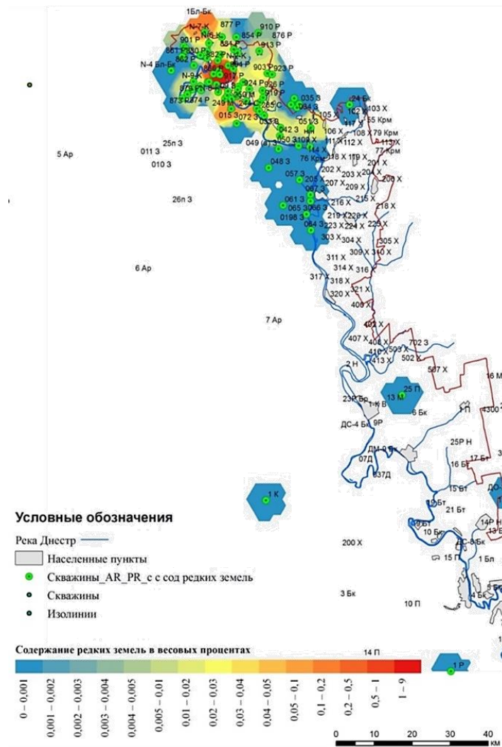
Рисунок 2 – Карта содержаний суммы редкоземельных элементов
