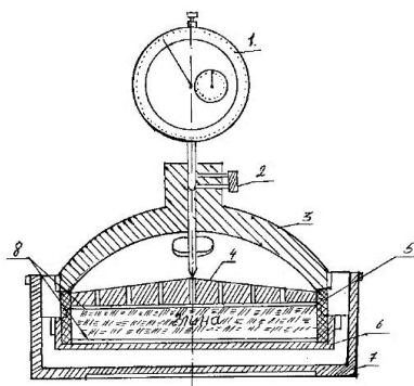
1 – индикатор часового типа; 2 – винт для закрепления индикатора; 3 – соединительная скоба; 4 – перфорированный поршень; 5 – закрепители скобы; 6 – перфорированное дно; 7 – ванночка; 8 – грунт
