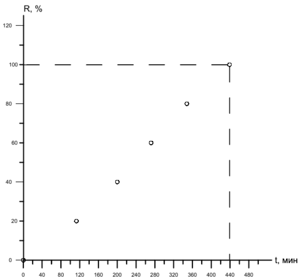
Рисунок 2 – Влияние нефтепродуктов на кинетику размокания глинистого грунта
