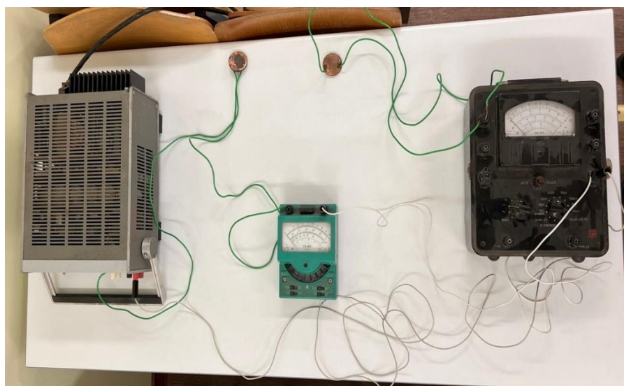
Рисунок 2 – Электрическая цепь
