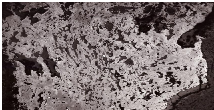
Рисунок 7 – Дендритоподобные выделения браннерита. Аншлиф. Скважина № 1449 – 278,0 м. Увеличение 200× Фото автора
