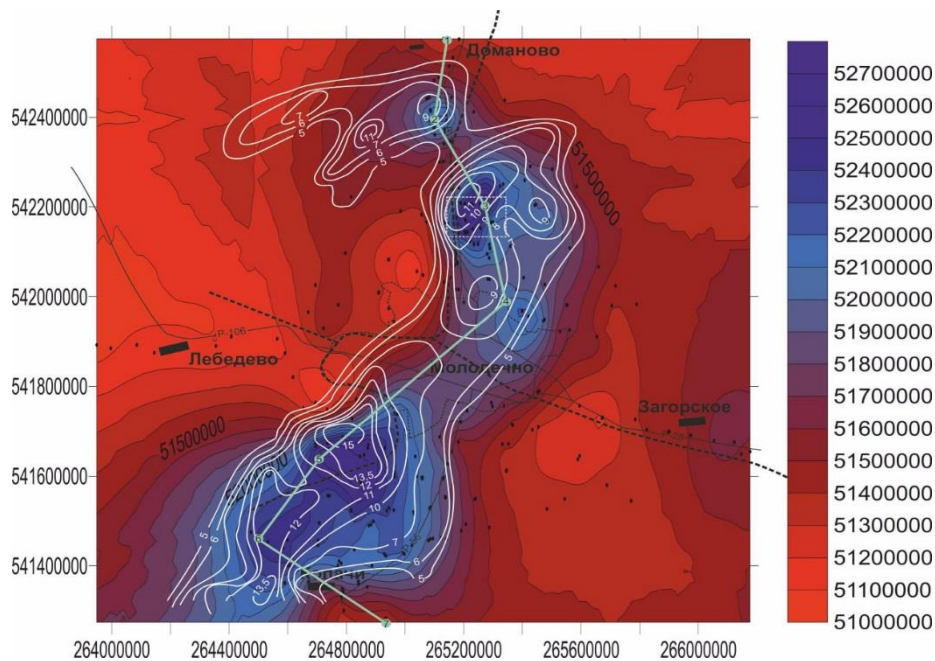
Рисунок 3 – Схема магнитных аномалий на участке Молодечненского геодинамического полигона
