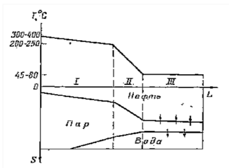
Рисунок 1 – Зоны, образующиеся при вытеснении нефти паром
