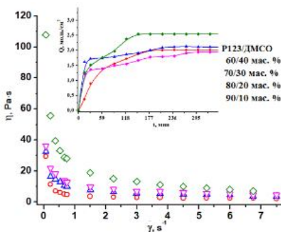
Рис.1 Кривые вязкости и высвобождения ибупрофена из ЛЖК систем P123®/ДМСО
