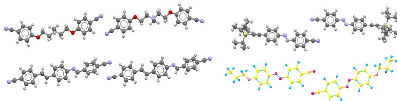
Рис. Строение ассоциатов производных бензонитрила: 1(а-в)– КБД, 1г – расчет ассоциата ФБ (B97D/6–311++G**)
