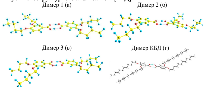
Рис. Строение 3,4-диАОБК: 1(а-в)– B97D/6-311G**, 1г – КБД
