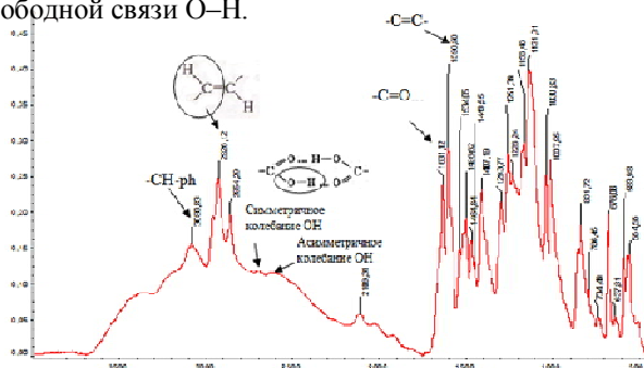
Рис. Экспериментальный ИК-спектр 4,4'-СДК
