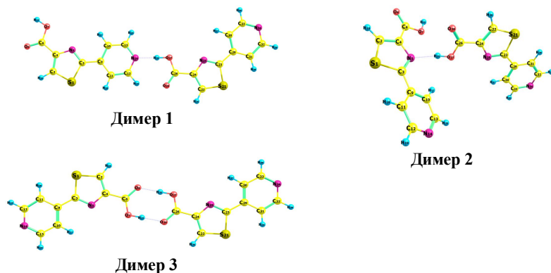
Рис. Геометрическое строение димеров молекулы PyTCA
