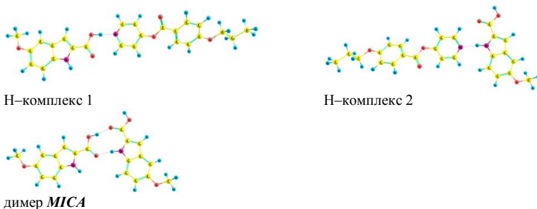
Рис. Геометрическое строение комплексов молекулы MICA
