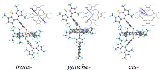
Рис. Геометрическое строение конформеров триады
