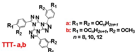
Рис. Исследуемые производные тристриазолтриазина
