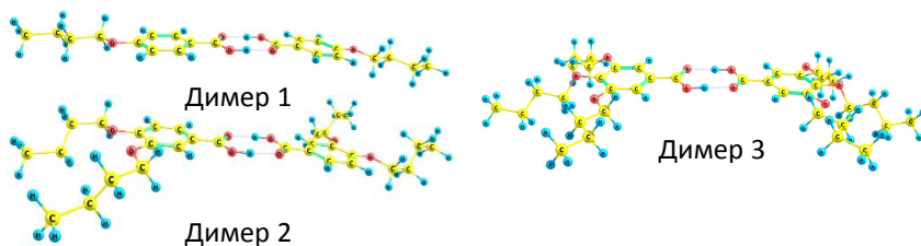
Рис. Димеры алкилоксибензойной кислоты
