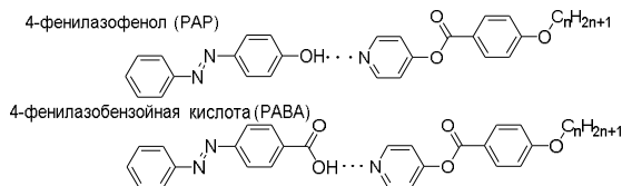
Рис. Структурные формулы исследуемых соединений и их Н-комплексов
