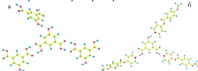
Рис. Строение тетрамера 5- ГИФК (а) и ее Н-комплекса с ПЭМОБК (б)
