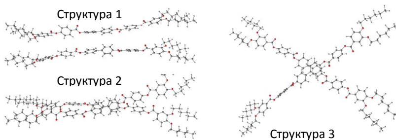
Рис. Оптимизированные структуры ассоциатов из двух молекул тетракатенарных мезогенов при разных вариантах самосборки
