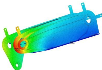
Рис. Карта напряжений при угле подъема стрелы 30 градусов
