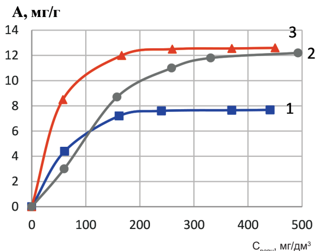
Рис. 3. Зависимость сорбционной емкости (A) образцов опилок от равновесной концентрации ионов меди(II) в растворе ( C_{равн} ): 1 – термообработанный образец 4; 2 – сорбент 5, термохимически модифицированный 5н HNO_3 ; 3 – сорбент 6, термохимически модифицированный 1%-м раствором лимонной кислоты
