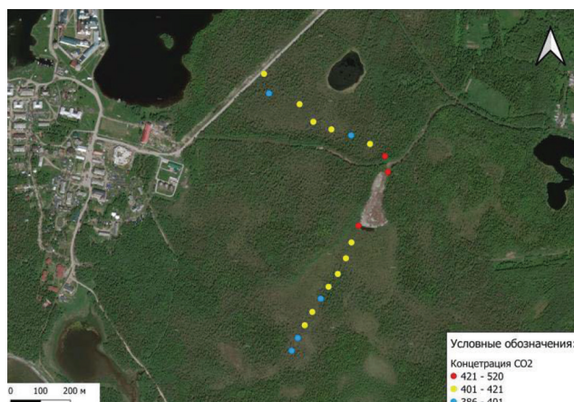
Рис. 5. Карта концентрации \text{CO}_2 (ppm) в атмосферном воздухе в радиусе 400 м к северо-западу и в 500 м к югу от полигона с шагом измерения 50 м
