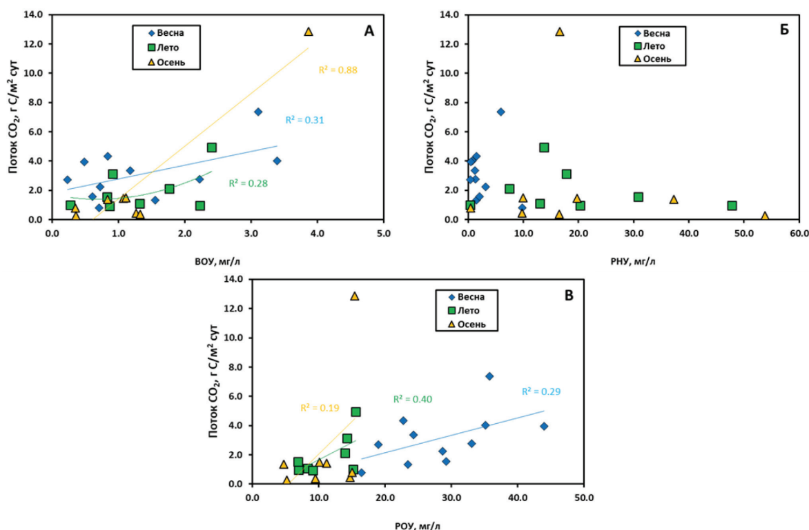
Рис. 2. Зависимость эмиссии \text{CO}_2 от концентрации ВОУ (А), РНУ (Б), РОУ (В)
