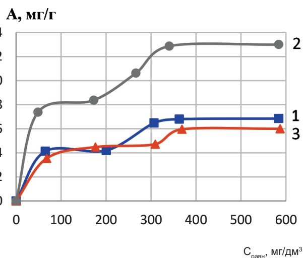
Рис. 2. Зависимость сорбционной емкости ( A ) образцов древесных опилок от равновесной концентрации ионов никеля(II) в растворе ( C_{\text{равн}} ): 1 – нативный образец 1; 2 – сорбент 2, химически модифицированный 5н \text{HNO}_3 ; 3 – сорбент 3, химически модифицированный 1%-м раствором лимонной кислоты
