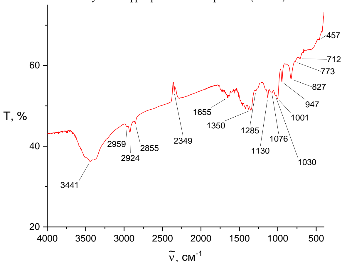
Рисунок 2. ИК-спектр образца сажи
