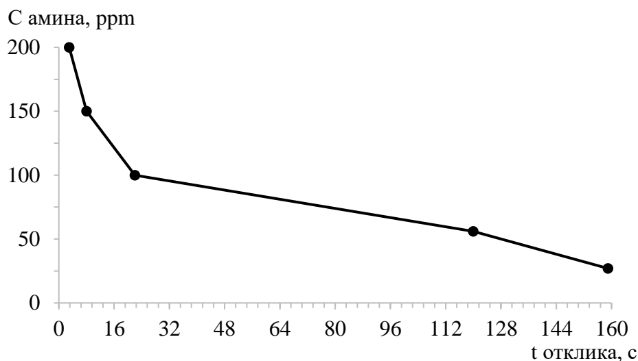
Рисунок 3. Зависимость времени отклика от концентрации монометиламина
