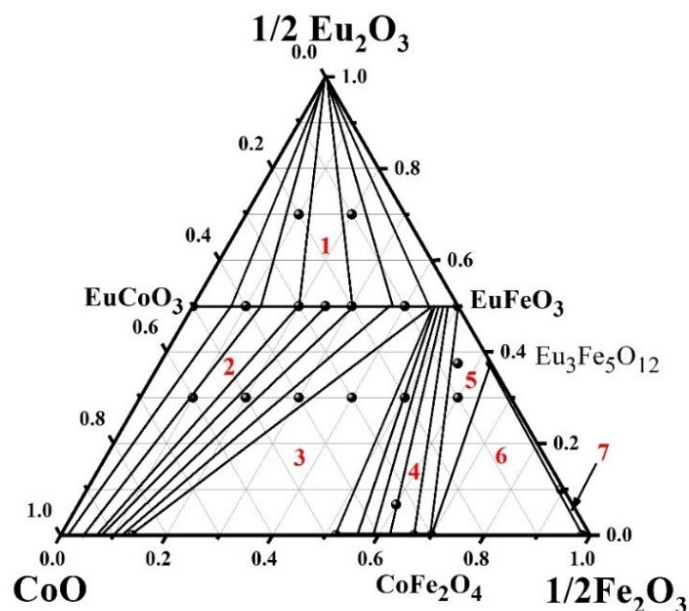
Рисунок 3. Изобарно-изотермический разрез диаграммы состояния системы \text{Eu}_2\text{O}_3\text{-Fe}_2\text{O}_3\text{-CoO} при 1100^\circ\text{C} на воздухе
