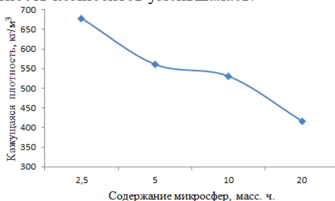
Рисунок 2. Зависимость плотности от содержания микросфер в образце
