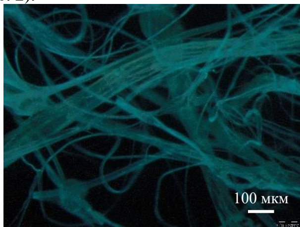
Рисунок 2. Микроволокна из поликарбоната, допированные \text{HODVMBF}_2 (2,5 мас. %) (снимок при облучении УФ светом, 254 нм)
