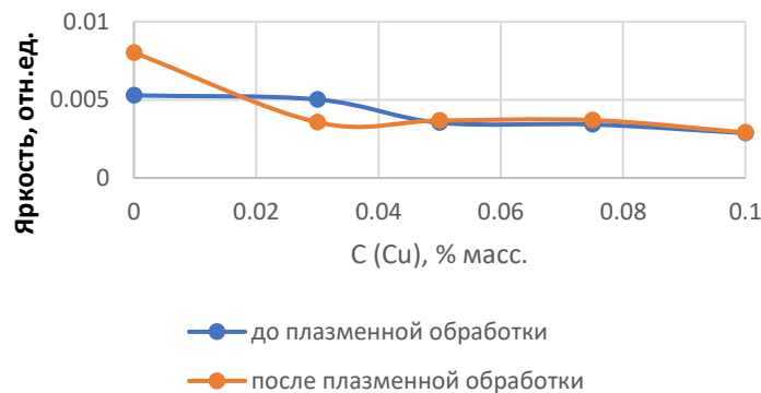
Рисунок 3. Яркость люминесценции при различных концентрациях активатора Cu
