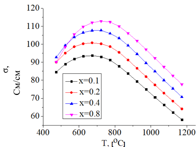
Рисунок 3. Температурная зависимость электропроводности ряда \text{La}_{2-x}\text{Sm}_x\text{NiO}_{4+\delta}
