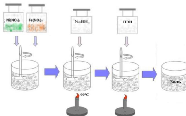
Рисунок 1. Схема синтеза феррита никеля в присутствии борогидрида натрия
