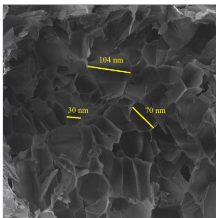
Рисунок 3. Микрофотография композиции, модифицированной триметилпропаном.
