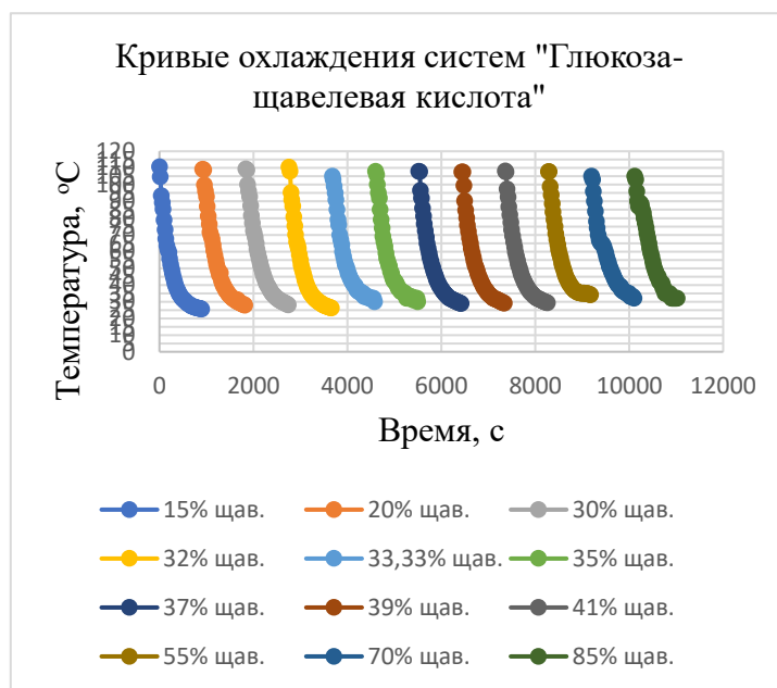
Рисунок 1. Кривые охлаждения системы «глюкоза – щавелевая кислота»
