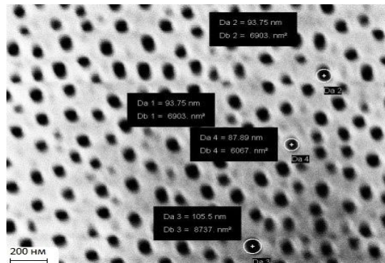
б) РЭМ-изображение ПАОА. Электролит на основе щавелевой кислоты
