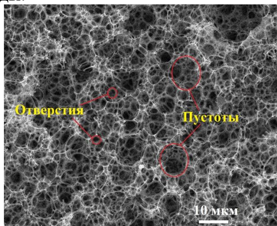
Рисунок 1. Микрофотография высокопористого сополимера стирола и дивинилбензола с составом исходной эмульсии: 90% воды и 0,5 об.% ПАВ
