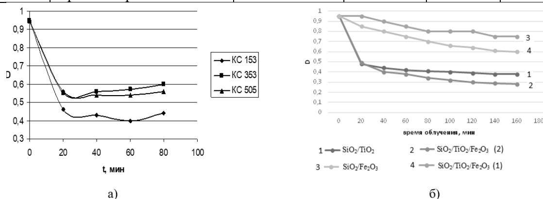
Рисунок 4. Зависимость оптической плотности раствора метиленового голубого от времени облучения
