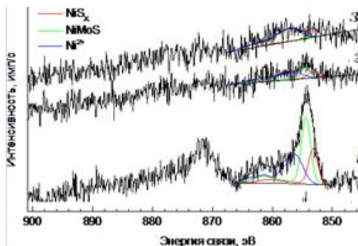
Рисунок 1. Ni2p РФЭС спектры исследованных образцов
