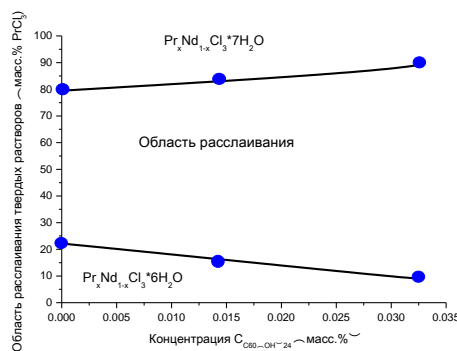
Рисунок 2. Диаграмма расщепления твердых растворов в четверной системе \text{C}_{60}(\text{OH})_{24} - \text{NdCl}_3 - \text{PrCl}_3 - \text{H}_2\text{O} при 25^\circ\text{C} : синие кружки – предельные составы расщепляющихся равновесных с жидким раствором твердых растворов (\text{PrCl}_3)_x(\text{NdCl}_3)_{1-x} \cdot 7\text{H}_2\text{O} и (\text{PrCl}_3)_x(\text{NdCl}_3)_{1-x} \cdot 6\text{H}_2\text{O} как функция содержания фуллеренола \text{C}_{60}(\text{OH})_{24} в растворе
