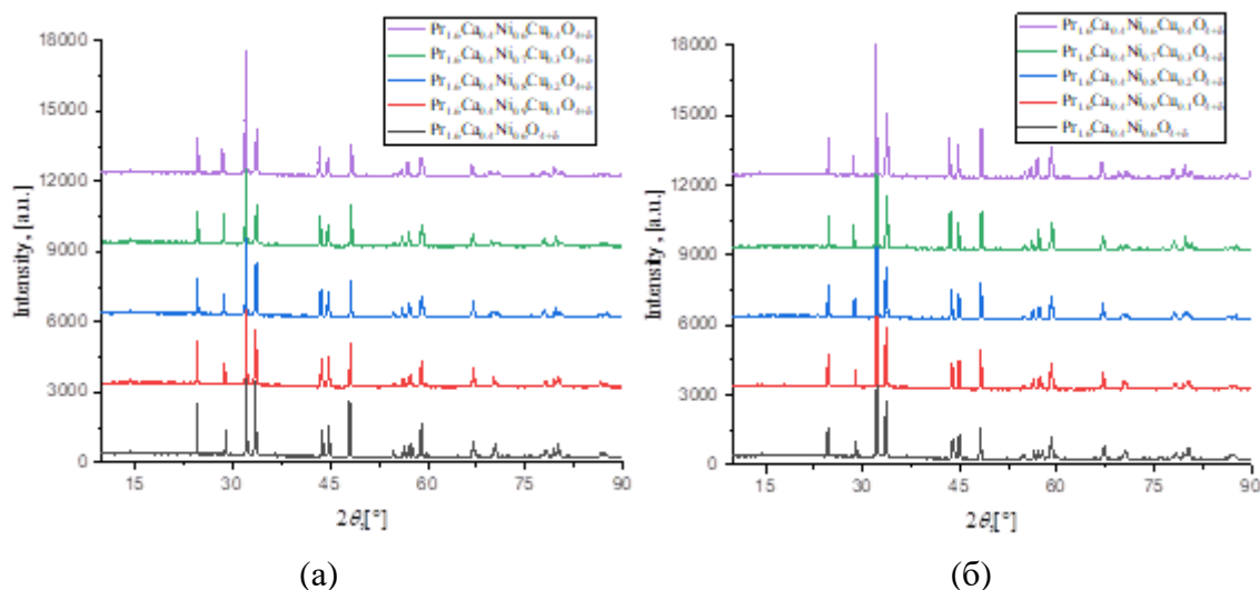
Рисунок 1. Порошковые рентгенограммы для \text{Pr}_{1.6}\text{Ca}_{0.4}\text{Ni}_{1-y}\text{Cu}_y\text{O}_{4+\delta} , полученных цитрат-нитратным (а) и полимер-нитратным (б) методами.
