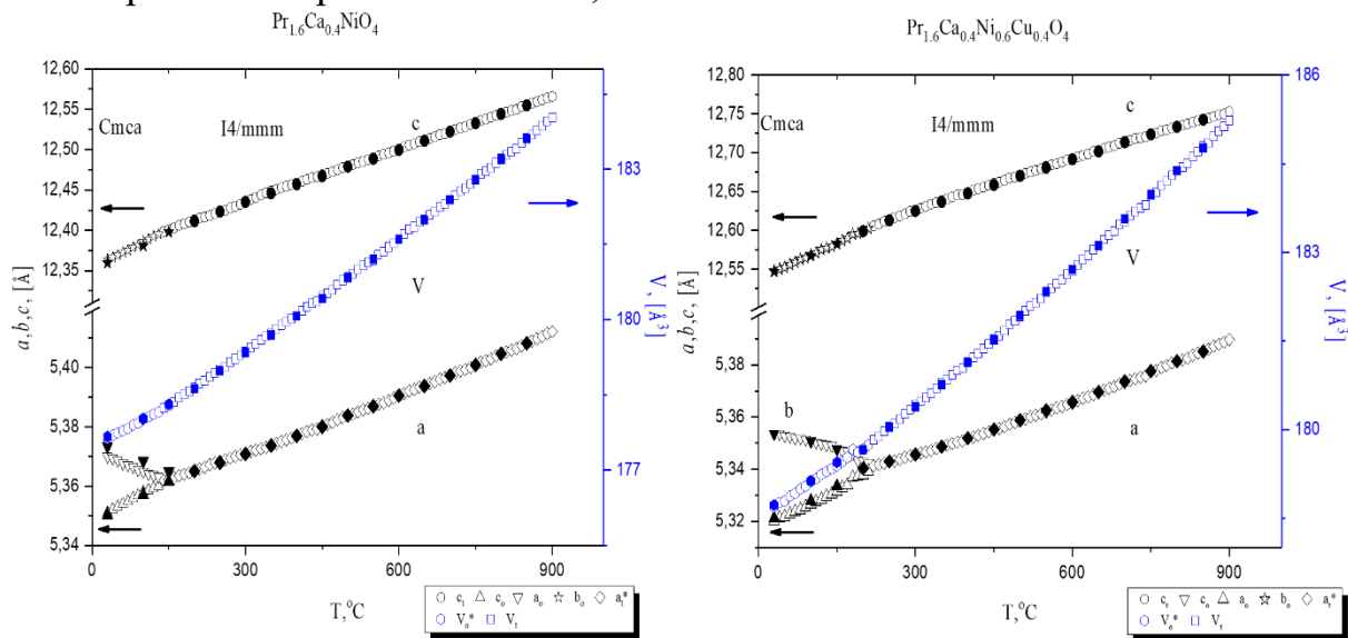
Рисунок 3. Температурные зависимости параметров и объема элементарных ячеек \text{Pr}_{1.6}\text{Ca}_{0.4}\text{Ni}_{1-y}\text{Cu}_y\text{O}_{4+\delta} ( y=0.0; 0.4 ), полученных цитрат-нитратным методом.
