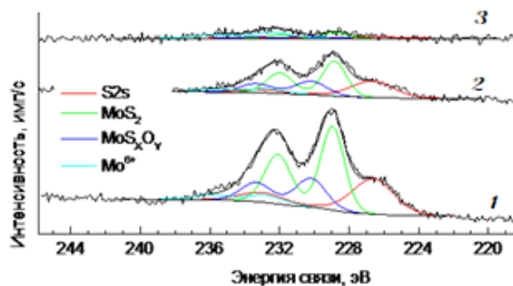
Рисунок 2. Mo3d и S2s РФЭС спектры исследованных образцов
