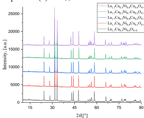
Рисунок 2. Порошковые рентгенограммы для \text{La}_{1.7}\text{Ca}_{0.3}\text{Ni}_{1-y}\text{Cu}_y\text{O}_{4+\delta} .
