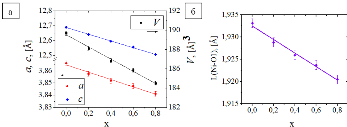
Рисунок 2. Концентрационные зависимости профильных и структурных параметров \text{La}_{2-x}\text{Sm}_x\text{NiO}_{4+\delta} : а) параметры и объем элементарной ячейки; б) межатомные расстояния Ni-O1
