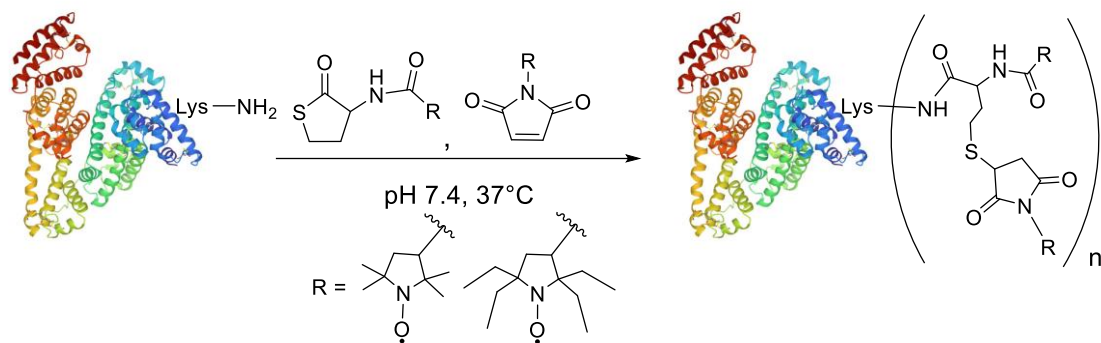
Рисунок 1. Синтез модифицированного HSA с нитроксильными радикалами
