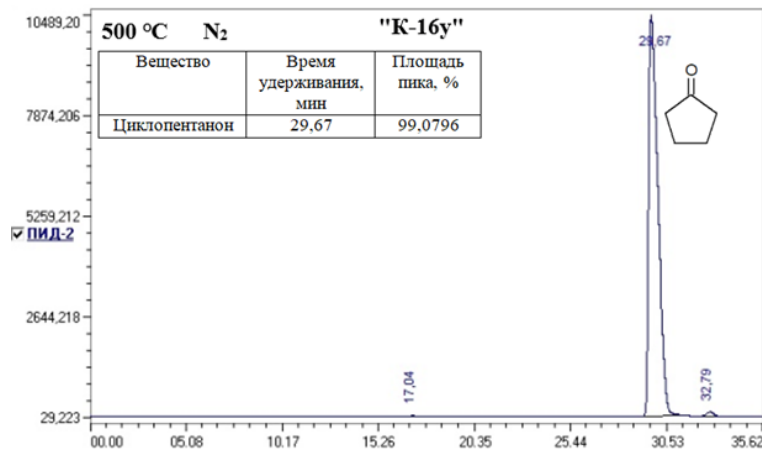
Рисунок 5. Хроматограмма продукта, полученного при 500 °С в атмосфере азота (4 часа)
