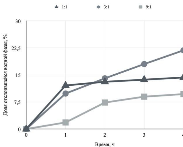
Рисунок 2. Зависимость доли отслоившейся водной фазы от времени
