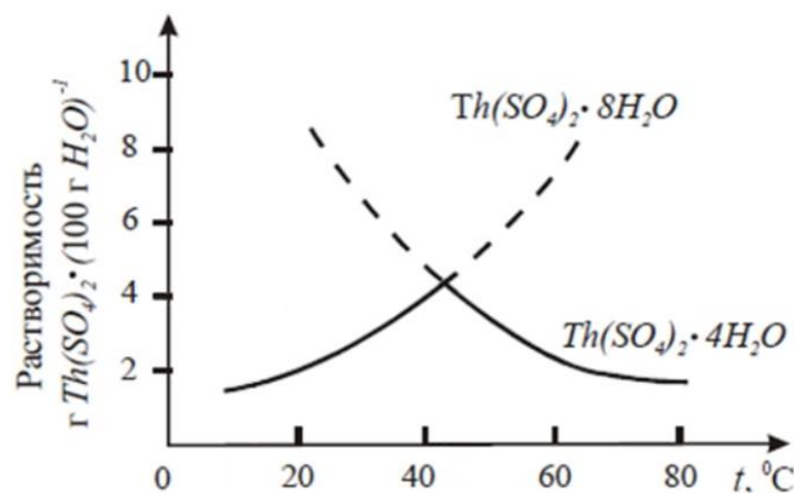
Рисунок 1. Зависимость растворимости сульфата тория от температуры [4].
