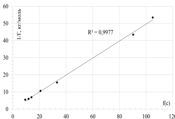
Рисунок 4. Линейная форма изотермы сорбции ионов церия из нитратных сред
