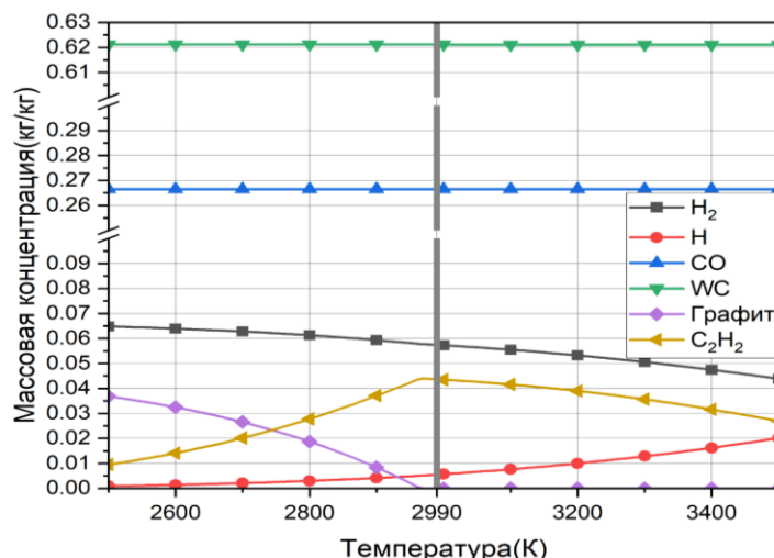
Рисунок 3. Зависимость концентрации продуктов реакции от температуры при удельном расходе метана 0,36 кг/кг оксида вольфрама
