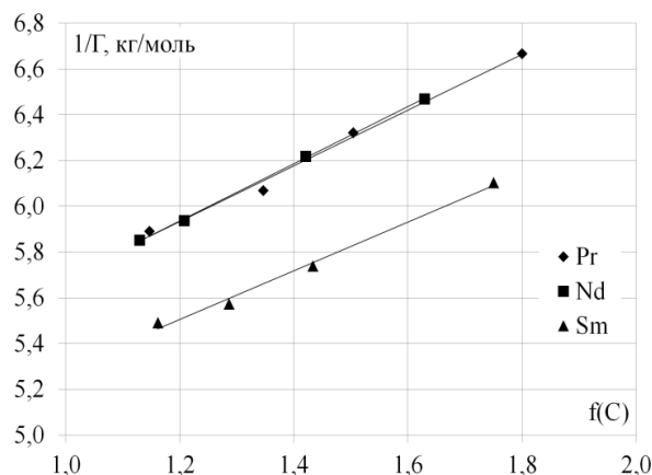
Рисунок 5. Линейные формы изотерм сорбции празеодима, неодима и самария из сульфатных сред
