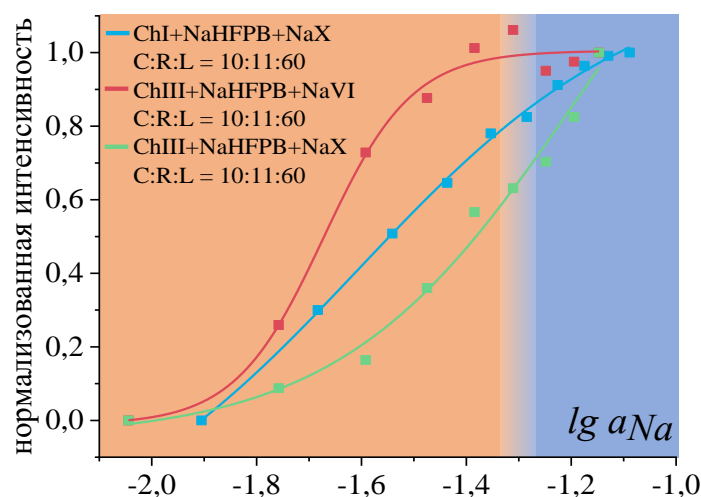
Рисунок 1. Градуировка натрий-селективных оптодных составов по модельным растворам пота, нормированная на единицу. Синяя кривая – «кислый» пот; красная кривая – «щелочной» пот; зеленая кривая – нейтральный стандарт. Коричневый диапазон – нормальная концентрация \text{Na}^+ в поте, синий – повышенная концентрация.
