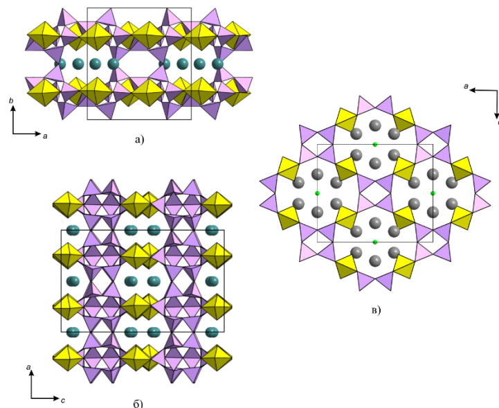
Рисунок 1. Проекция кристаллографических структур соединений \text{Rb}_2(\text{UO}_2)_2(\text{Si}_5\text{O}_{13})(\text{H}_2\text{O})_2 (а), \text{Rb}_2(\text{UO}_2)_2(\text{Si}_8\text{O}_{19})(\text{H}_2\text{O})_4 (б) и \text{Cs}_3\text{Cl}(\text{UO}_2)(\text{Si}_4\text{O}_{10}) (в). Полиэдры урана показаны желтым цветом, кремния – сиреневым, темно-зеленые атомы рубидия, серые – цезия, зеленые – хлора, молекулы воды, расположенные в полостях каркасов, убраны с проекций.
