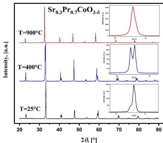
Рисунок 1. Рентгенограммы \text{Sr}_{0.3}\text{Pr}_{0.7}\text{CoO}_{3-\delta} при 25°C, 400°C, 900°C
