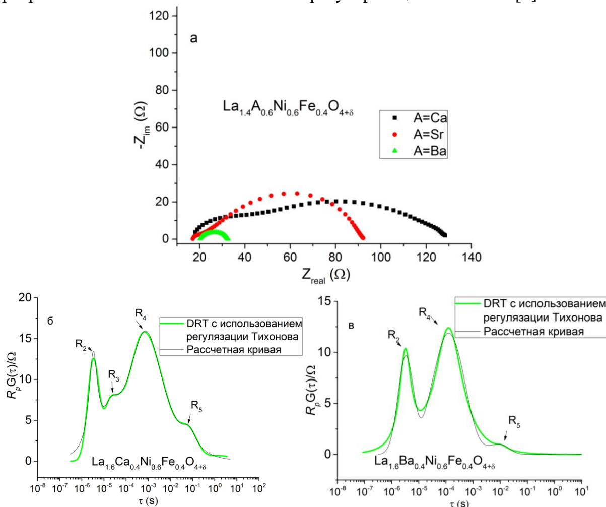
Рисунок 1. Годографы импеданса симметричных ячеек LANF0604 (A=Ca, Sr, Ba)/SDC (а), функция DRT при 800 °С для симметричной ячейки LCNF0604/SDC (б), функция DRT при 700 °С для симметричной ячейки LBNF0604/SDC (в)
