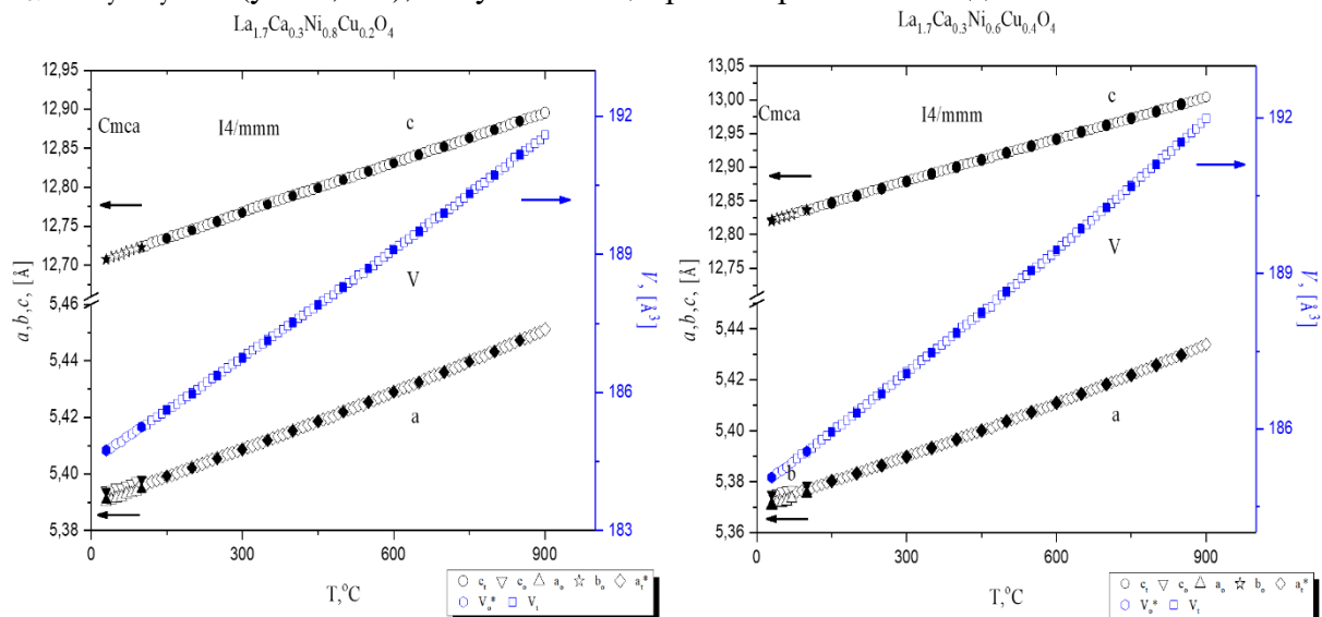
Рисунок 4. Температурные зависимости параметров и объема элементарных ячеек \text{La}_{1.7}\text{Ca}_{0.3}\text{Ni}_{1-y}\text{Cu}_y\text{O}_{4+\delta} ( y=0.2; 0.4 ).
