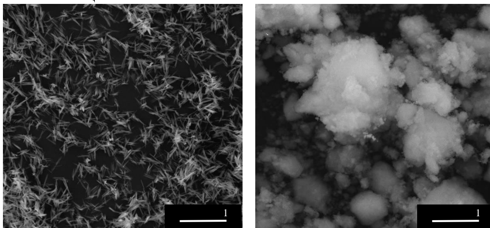
Рисунок 2. Снимки СЭМ частиц: а) образца Gd_{0,5}Y_{0,5}PO_4 со структурой рабдофана; б) образца YPO_4 со структурой ксенотима
