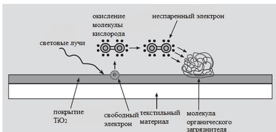
Рисунок 1. Механизм самоочищения хлопчатобумажной ткани с наночастицами диоксида титана
