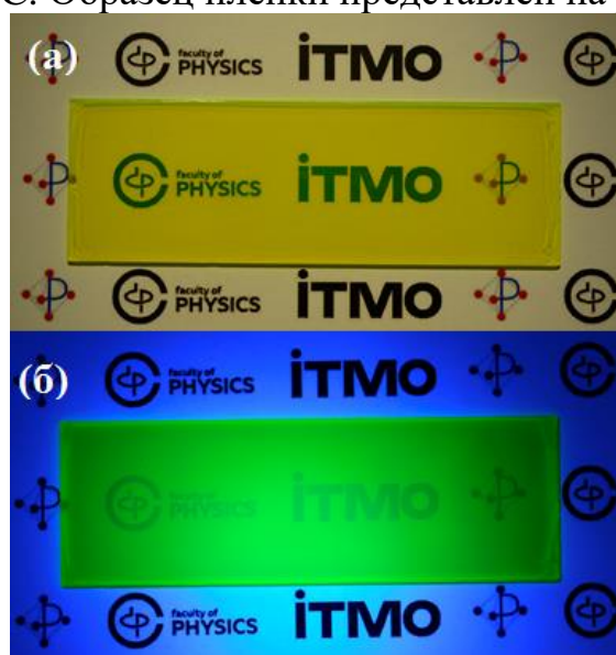
Рисунок 3. Образец пленки из нанокристаллов CsPbBr 3 , полученной ракельным нанесением на поверхности гидрофобизированной стеклянной подложки, при видимом (а) и ультрафиолетовом (б) освещении
