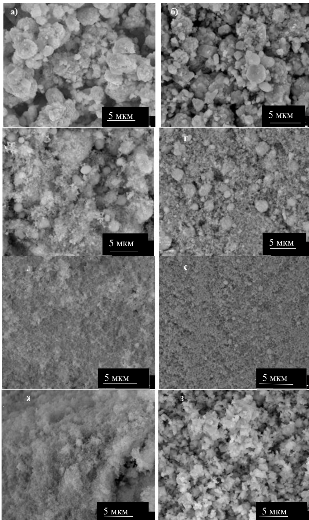
Рисунок 3. \text{BiVO}_4 до (а) и после (б) ГТС, \text{BiP}_{0,8}\text{V}_{0,2}\text{O}_4 до (в) и после (г) ГТС, \text{BiP}_{0,5}\text{V}_{0,5}\text{O}_4 до (д) и после (е) ГТС, \text{BiPO}_4 до (ж) и после(з) ГТС
