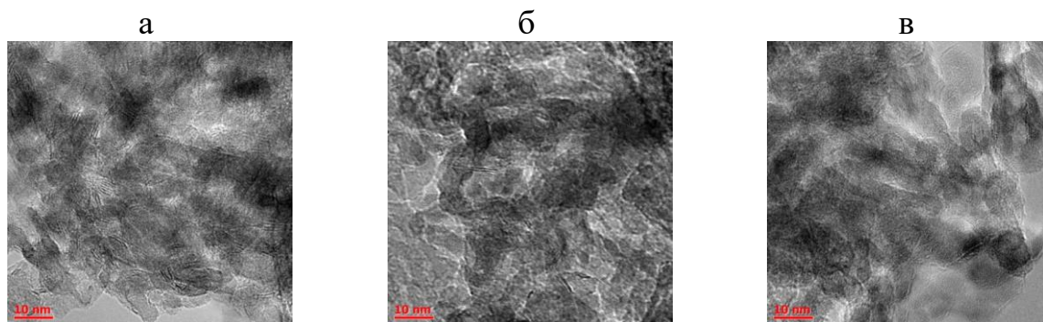
Рисунок 3. Изображения образцов ПЭМ ВР образца №1 (а), образца №2 (б), образца №3 (в).
