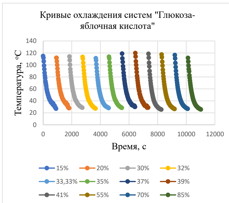
Рисунок 2. Кривые охлаждения системы «глюкоза – яблочная кислота»
