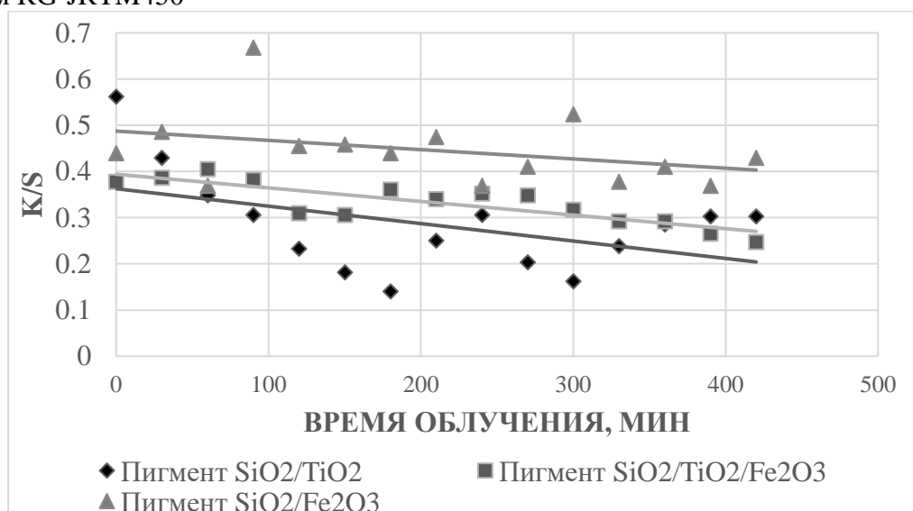
Рисунок 5. Зависимость интенсивности окраски от времени облучения образцов со связующим Astronal 9014
