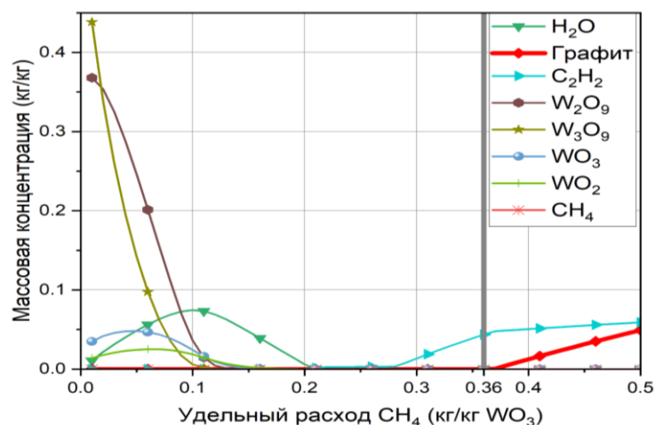
Рисунок 2. Зависимость концентрации примесных продуктов реакции от удельного расхода метана при T=2990K
