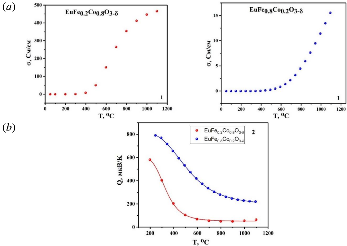
Рисунок 4. Температурные зависимости общей электропроводности \sigma (a) и коэффициента Зеебека (b) для сложных оксидов \text{EuFe}_{0.2}\text{Co}_{0.8}\text{O}_{3-\delta} и \text{EuFe}_{0.8}\text{Co}_{0.2}\text{O}_{3-\delta}
