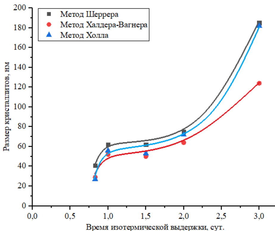
Рисунок 3. Зависимость размеров кристаллитов соединения со структурой вейлендита от продолжительности изотермической выдержки в гидротермальных условиях при pH=5
