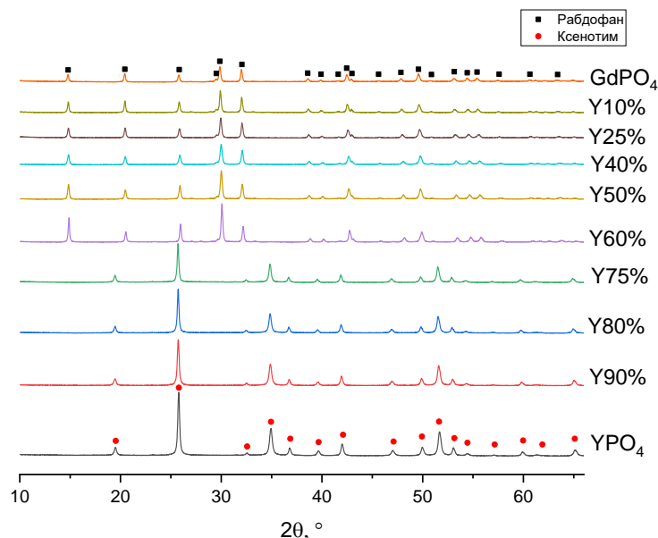
Рисунок 1. Дифрактограммы образцов Gd_{1-x}Y_xPO_4 \cdot nH_2O после ГТО при T=230^\circ C и \tau=2h . Анализ порошковых дифрактограмм показал, что образцы Gd_{1-x}Y_xPO_4 \cdot nH_2O , полученные гидротермальным методом, образуют твердые растворы как для структуры рабдофана, так и ксенотима, на что указывают практически линейные зависимости параметров элементарной ячейки от состава.
