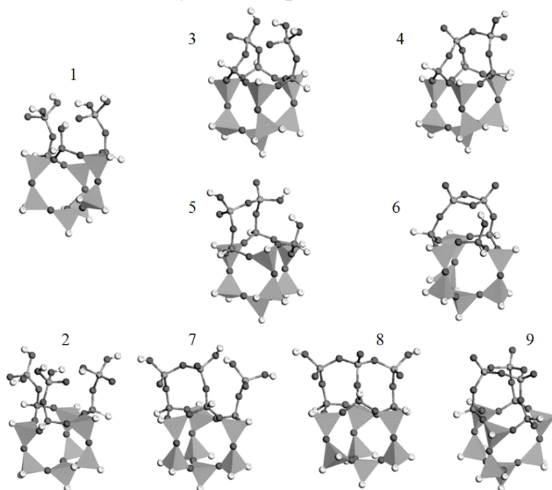
Рисунок 1. Кластерные модели поверхности кремнезема с двумя (1) либо тремя (2) изолированными монофункциональными ванадийгидроксидными группами и возможные продукты их конденсации при протекании вторичных химических превращений (3-9)
