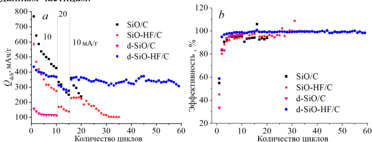
Рисунок 1. Зависимость разрядной емкости (а) и кулоновской эффективности (б) от номера цикла
