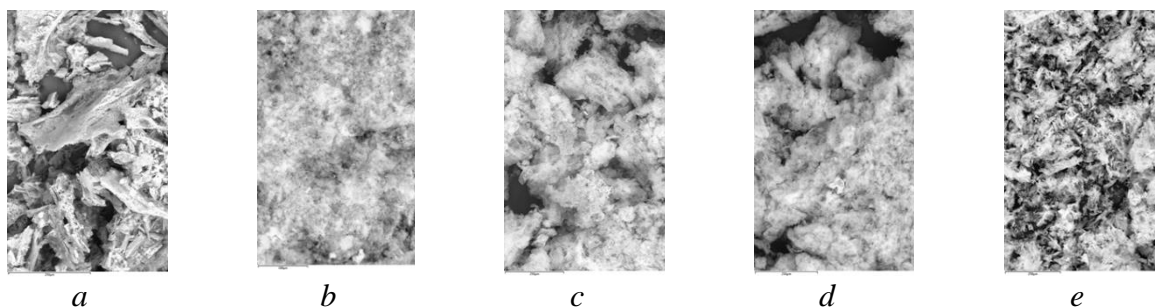
Рисунок 2. СЭМ образцов, синтезированных при N/G=1/1 и соотношениях Al/Cr: 1/0 (a), 3/1 (b), 1/1 (c), 1/3 (d) и 0/1 (e), полученные при увеличении 250 нм (a,c,d,e) и 100 нм
