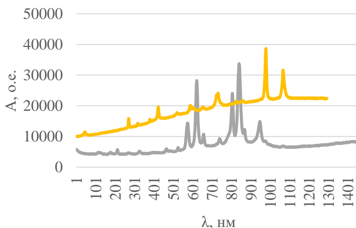
Рисунок 2. Обнаружение эффекта ГКР света на ТМ с осажденными НЧ серебра. Желтая линия – исходная ТМ ПЭТФ; серая линия – ТМ с осажденными НЧ серебра.
