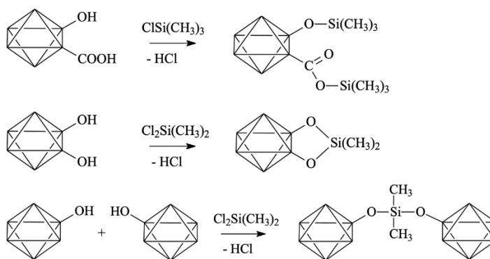
Рисунок 1. Схемы поверхностных модификаций ДНА
