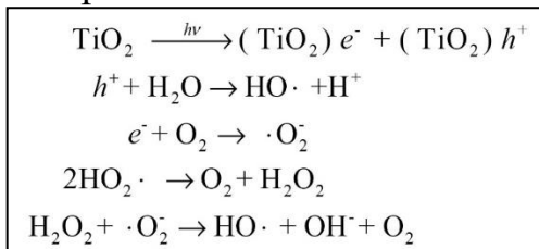
Рисунок 2. Реакции, протекающие на поверхности \text{TiO}_2 при окислении органических соединений
