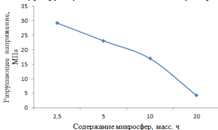
Рисунок 3. Зависимость разрушающего напряжения при сжатии от содержания микросфер в образце
