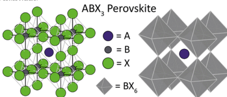
Рисунок 1. Стандартная структура кубического перовскита [1]
