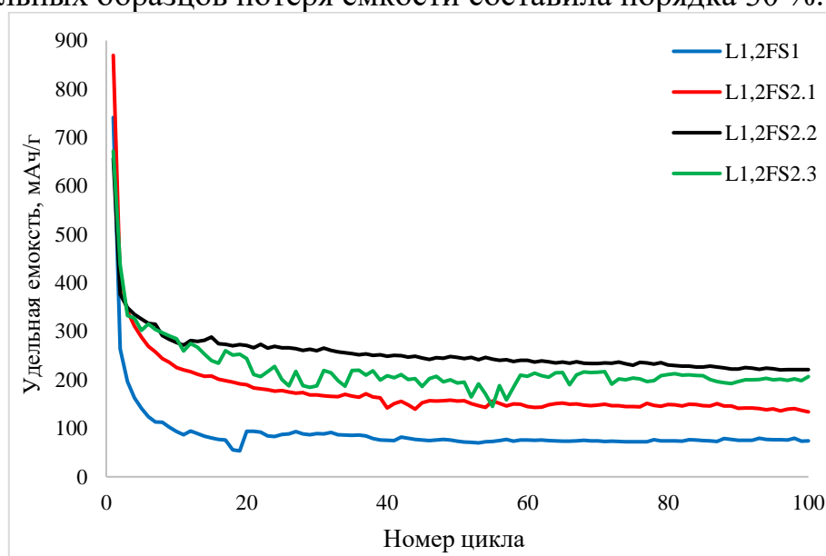
Рисунок 1. Циклическая стабильность образцов L 1,2 FS1 и L 1,2 FS2
