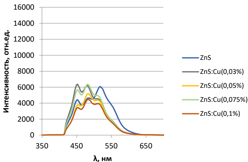
Рисунок 2. Спектр люминесценции люминофоров ZnS:Cu,Br для серии из модифицированной шихты
