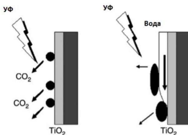
Рисунок 1. Схематичное представление процесса удаления загрязнений на самоочищающихся покрытиях
