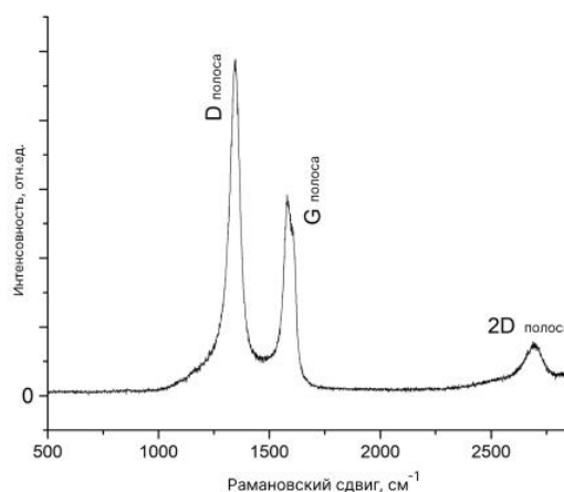
Рисунок 2. Спектр комбинационного рассеяния МГ
