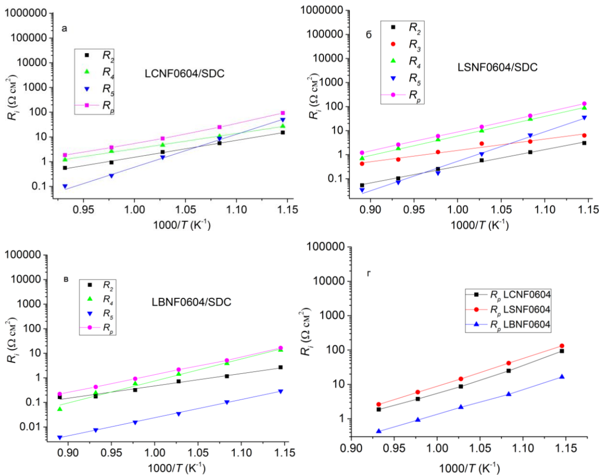
Рисунок 2. Температурные зависимости сопротивлений вкладов и общего поляризационного сопротивления симметричных ячеек LCNF0604/SDC (а), LSNF0604/SDC (б), LBNF0604/SDC (в), температурная зависимость общего поляризационного сопротивления для всех ячеек (г)
