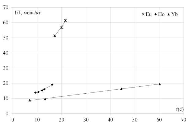
Рисунок 7. Линейные формы изотерм сорбции европия, гольмия и иттербия из фосфорнокислых сред на сорбенте, иммобилизованном Д2ЭГФК
