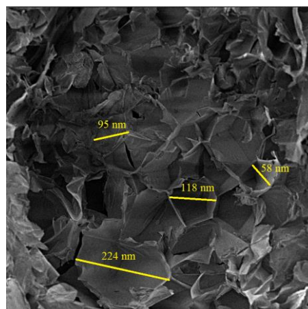
Рисунок 4. Микрофотография композиции, модифицированной полиэтиленгликолем.
