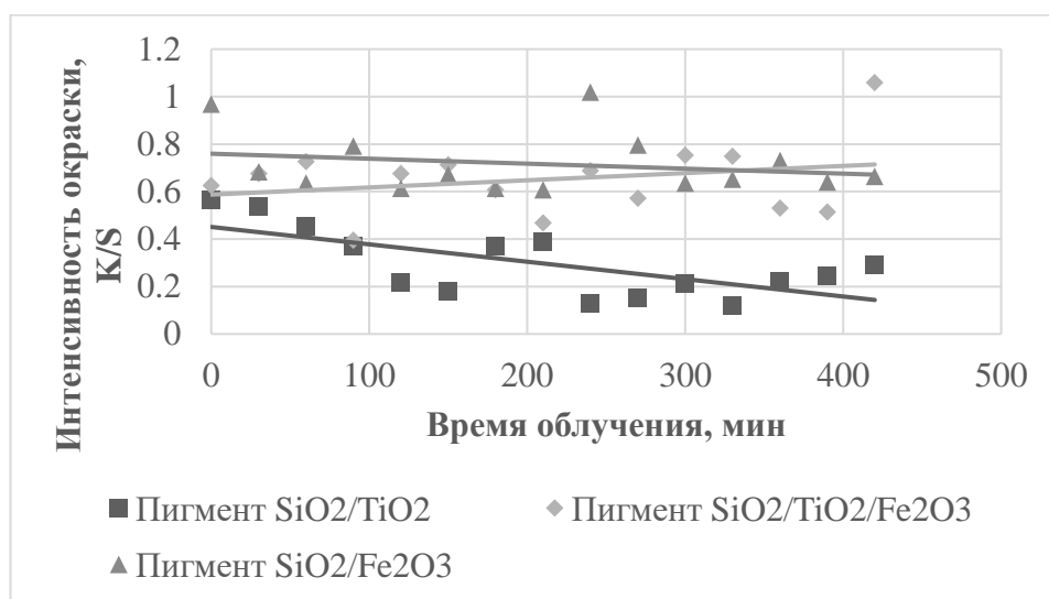
Рисунок 4. Зависимость интенсивности окраски от времени облучения образцов со связующим RG-JRTM450
