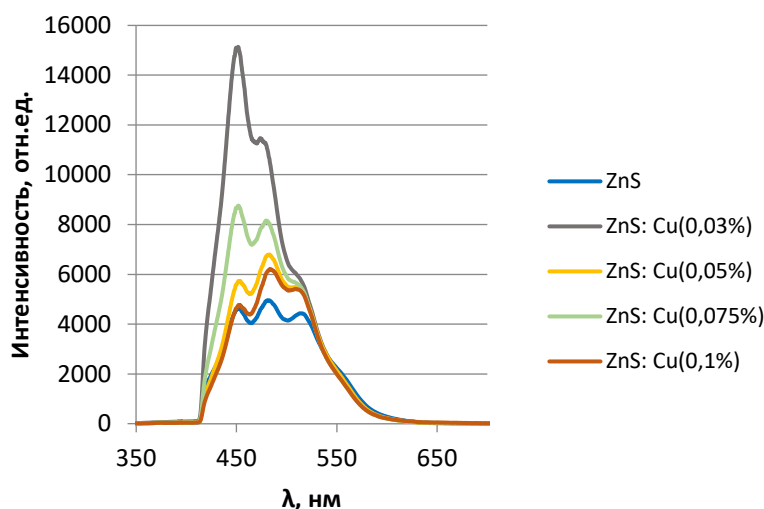
Рисунок 1. Спектр люминесценции люминофоров ZnS:Cu,Br для серии из немодифицированной шихты
