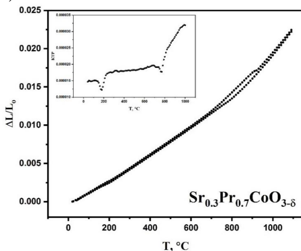
Рисунок 2. Зависимости относительного линейного расширения и КТР для \text{Sr}_{0.3}\text{Pr}_{0.7}\text{CoO}_{3-\delta} от температуры на воздухе
