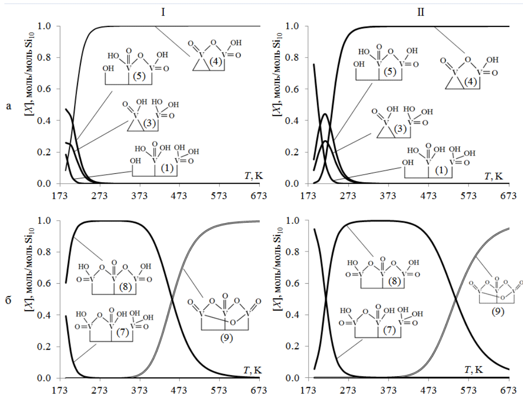
Рисунок 2. Расчетный прогноз состава продуктов взаимодействий между OH-группами, связанными с атомами ванадия в структурах исходной конфигурации 1 (а) и 2 (б) в отсутствие (I) и в присутствии (II) паров воды (парциальное давление 23.77 кПа) в системе в начальном состоянии. Числа в скобках соответствуют номеру конфигурации поверхностных центров на рисунке 1.
