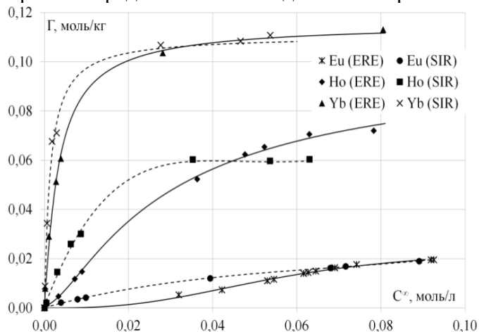
Рисунок 3. Экспериментальные формы изотерм сорбции европия, гольмия и иттербия на полимерных материалах, импрегнированных и иммобилизированных ди-2-этилгексилфосфорной кислотой
