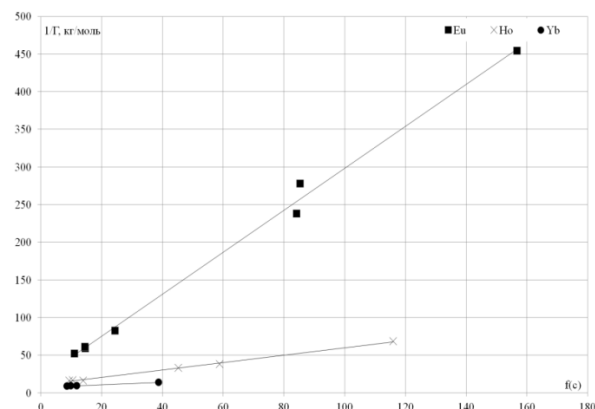
Рисунок 6. Линейные формы изотерм сорбции европия, гольмия и иттербия из фосфорнокислых сред на сорбенте, импрегнированном Д2ЭГФК
