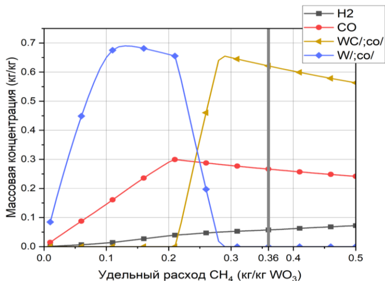
Рисунок 1. Зависимость концентрации основных продуктов реакции от удельного расхода метана при T=2990K
