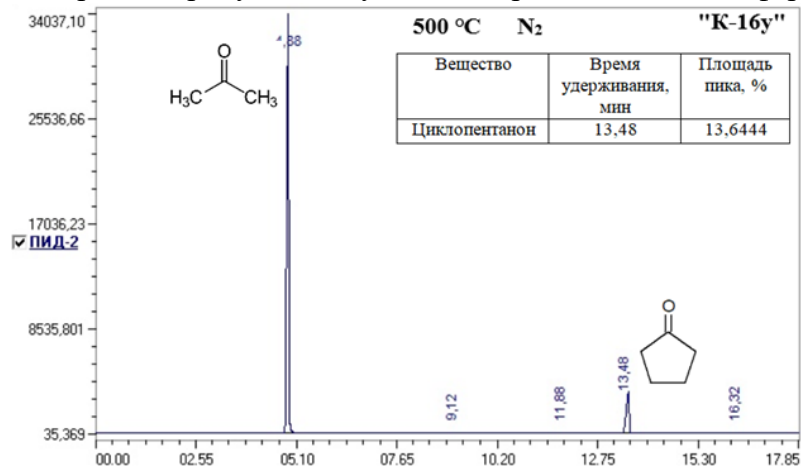
Рисунок 6. Хроматограмма продукта, полученного при 500 °С в атмосфере азота (4 часа)
