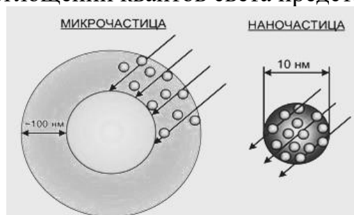
Рисунок 3. Поглощение квантов света в микро- и наночастицах
