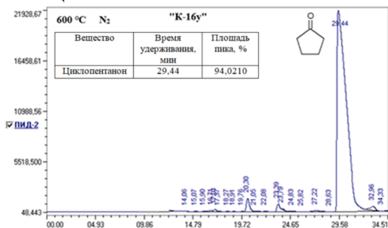
Рисунок 1. Хроматограмма продукта, полученного при 600 °С в воздушно-углеводородной атмосфере
