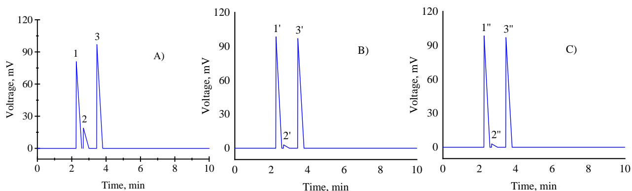
Рисунок 1. Хроматограммы реакционных растворов после окисления изопропанола (А), пропанола (В) и этанола (С)
