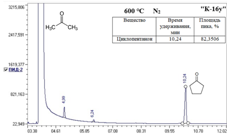
Рисунок 4. Хроматограмма продукта, полученного при 600 °С в атмосфере азота (4 часа)
