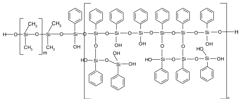
Рисунок 1. Блок-сополимер полидиметилсилоксан-полифенилсилсесквиоксан (ПДМС-ПФССО)
