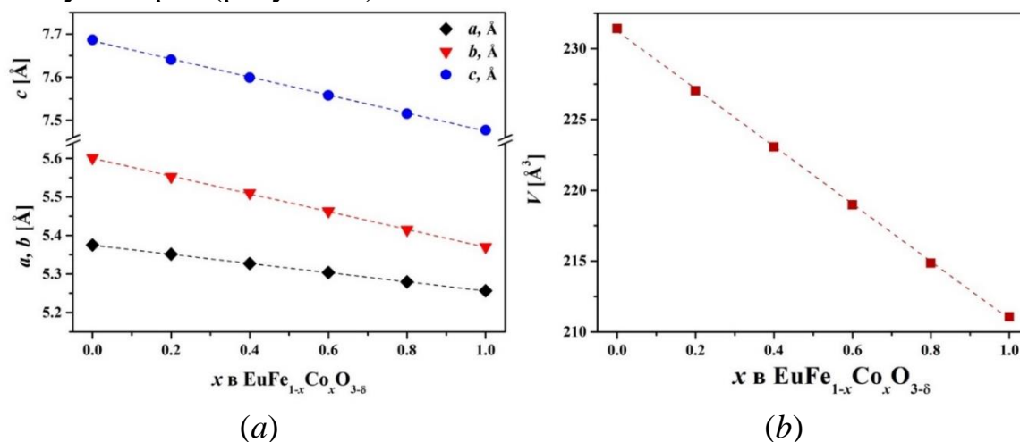
Рисунок 2. Зависимости параметров (a) и объёма (b) элементарной ячейки оксида от состава твёрдого раствора \text{EuFe}_{1-x}\text{Co}_x\text{O}_{3-\delta}
