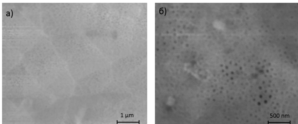
Рисунок 1. Микрофотографии образцов полученных при 80В и 15°С в а) 1М сульфат аммония; б) 100% глицерин
