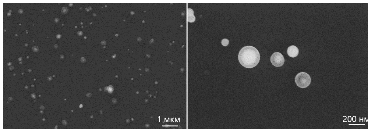
Рисунок 1. СЭМ-изображения композитных наночастиц образца №6
