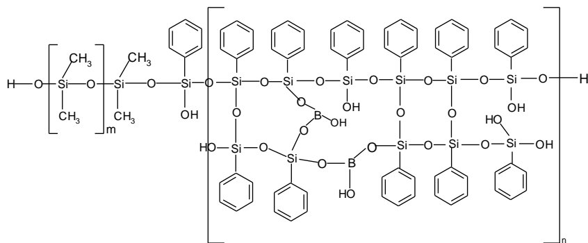
Рисунок 3. Предполагаемая структура полимера после модификации
