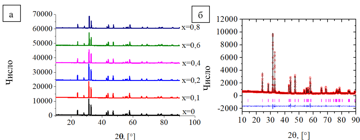
Рисунок 1. Данные рентгеновской порошковой дифракции: а) экспериментальные рентгенограммы ряда \text{La}_{2-x}\text{Sm}_x\text{NiO}_{4+\delta} ; б) экспериментальный и расчетный профили состава \text{La}_{1.6}\text{Sm}_{0.4}\text{NiO}_{4+\delta}
