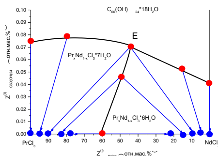
Рисунок 1. Диаграмма растворимости четверной системы NdCl 3 – PrCl 3 – C 60 (OH) 24 – H 2 O при 25°C: красные кружки – экспериментальные данные по составам насыщенных растворов, синие кружки – составы равновесных твердых растворов (PrCl 3 ) x (NdCl 3 ) 1-x · 7H 2 O и (PrCl 3 ) x (NdCl 3 ) 1-x · 6H 2 O; красная нонвариантная точка E (эвтоника); синими стрелками представлены ноды: жидкий раствор-твердый раствор 1 и жидкий раствор-твердый раствор 2 . Диаграммы представлены в индексах Йенеке растворенных компонентов (в безводных проекциях): Z_{PrCl_3} = \frac{C_{PrCl_3}}{C_{PrCl_3} + C_{NdCl_3} + C_{C_{60}(OH)_{24}}} * 100\% , Z_{NdCl_3} =
