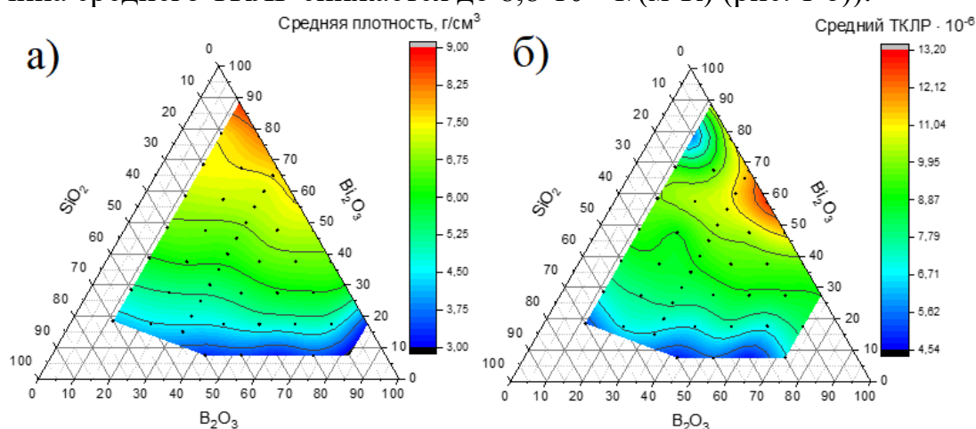
Рисунок 1. Изменение физико-химических свойств от состава: а – плотности, \text{г/см}^3 ; б – среднего ТКЛР, \text{1/(м}\cdot\text{К)} .
