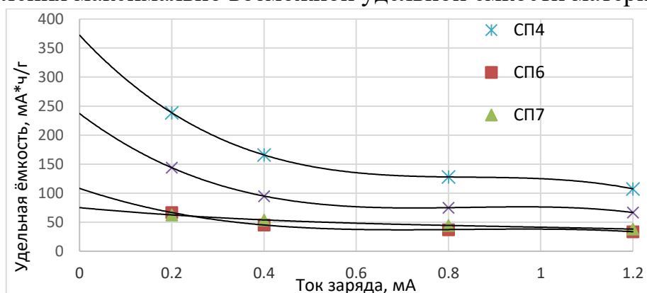
Рисунок 1. Зависимость удельной ёмкости от тока заряда
