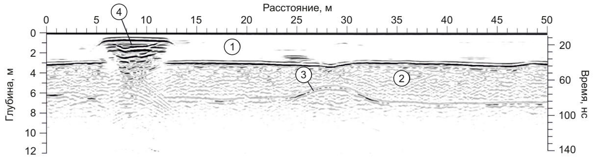
Рис. 11. Радарограмма по одному из профилей площадки № 2: 1 – лед; 2 – аллювий мерзлый; 3 – граница промерзания; 4 – локальная аномалия внутри льда.
