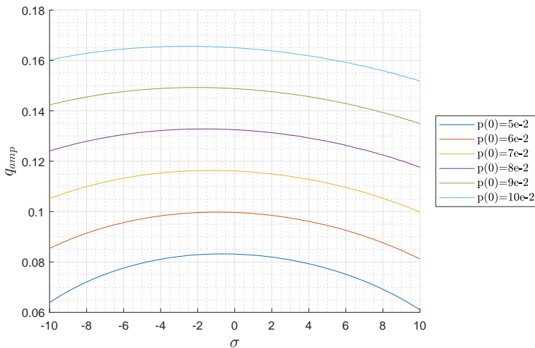
Рис. 16. Зависимость амплитуды второй рассматриваемой изгибной формы колебаний от частотной расстройки \sigma .
