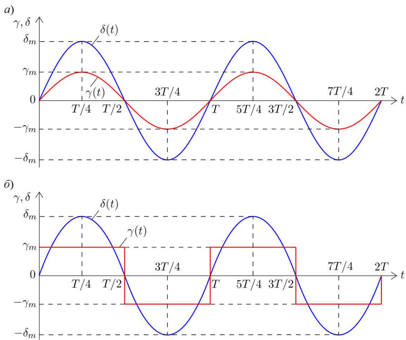
Рис. 6. Законы управления движением скейтборда: а – синусоидальный; б – скачкообразно-параболический
