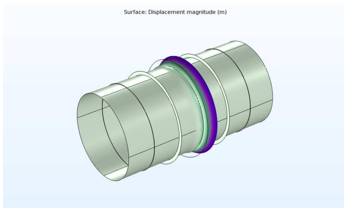
Рис. 6. «Пластинчатая» форма колебаний цилиндрической оболочки толщиной h = 0,01 , длиной l = 4 , подкрепленная пятью шпангоутами для случая линейной функции распределения с u = 8
