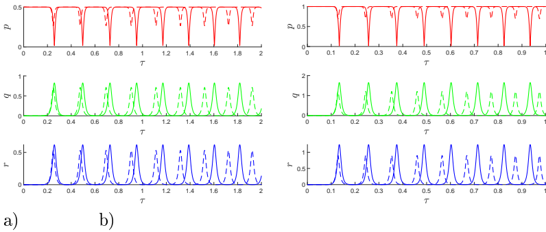
Рис. 13. Эволюция модальных амплитуд. Второе приближение — сплошная линия, третье — пунктирная линия для а) p(0) = 0.5 , б) p(0) = 1 .
