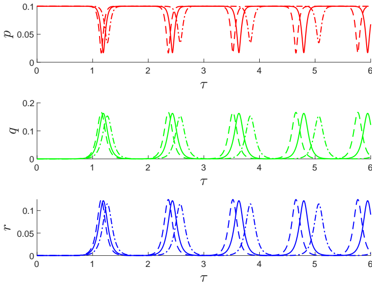
Рис. 9. Эволюция модальных амплитуд. \sigma = 5 — сплошная линия, \sigma = -5 — пунктирная линия, \sigma = 10 — штрих-пунктирная линия
