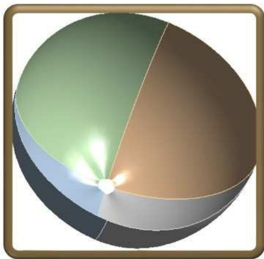
Рис. 3. Полусфера с возмущенной срединной поверхностью
