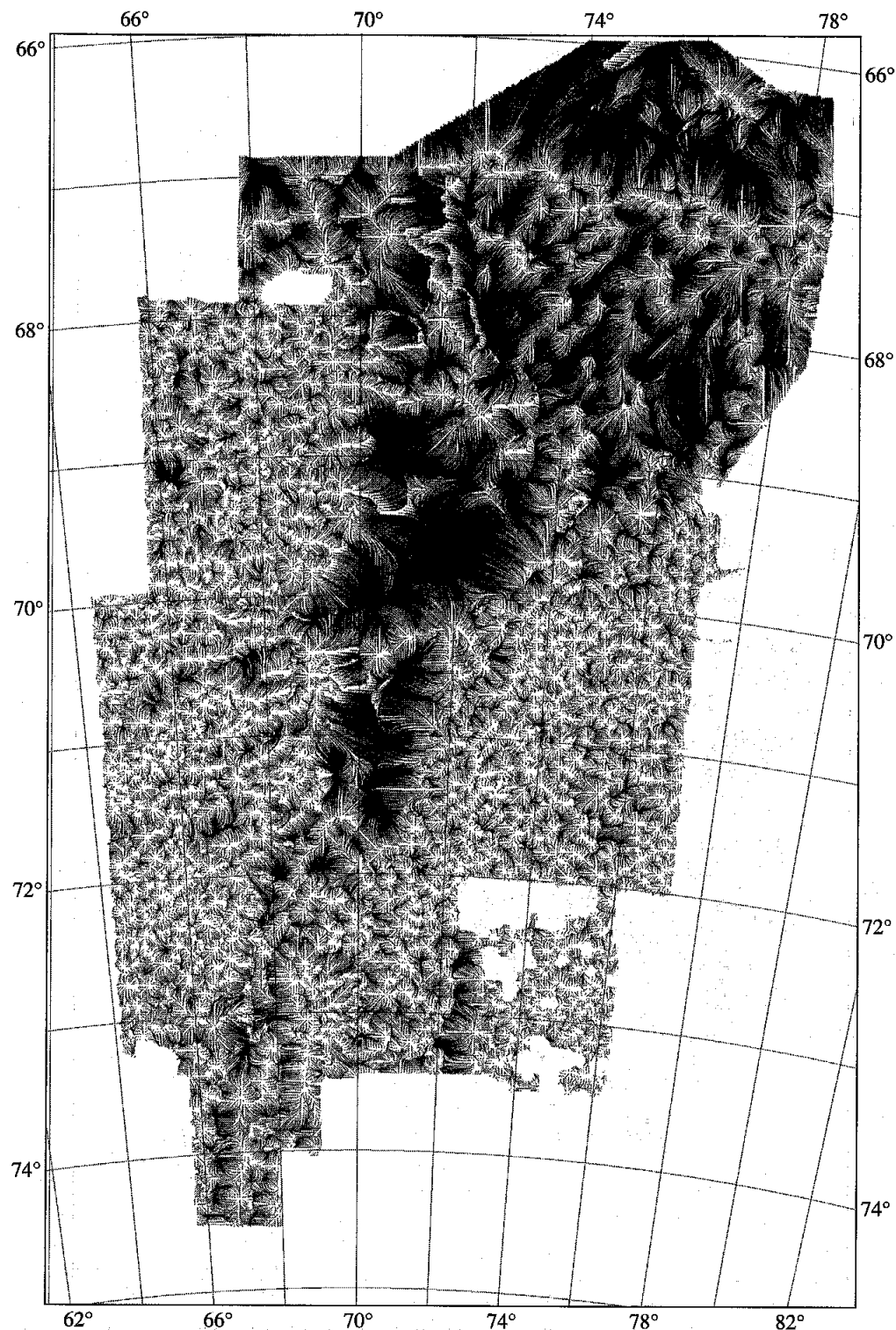
Рис. 4. Карта векторных линий подледно-подводной поверхности района грабена Ламберта (Восточная Антарктика) Линии тока и их сгущения показаны зонами различной насыщенности
