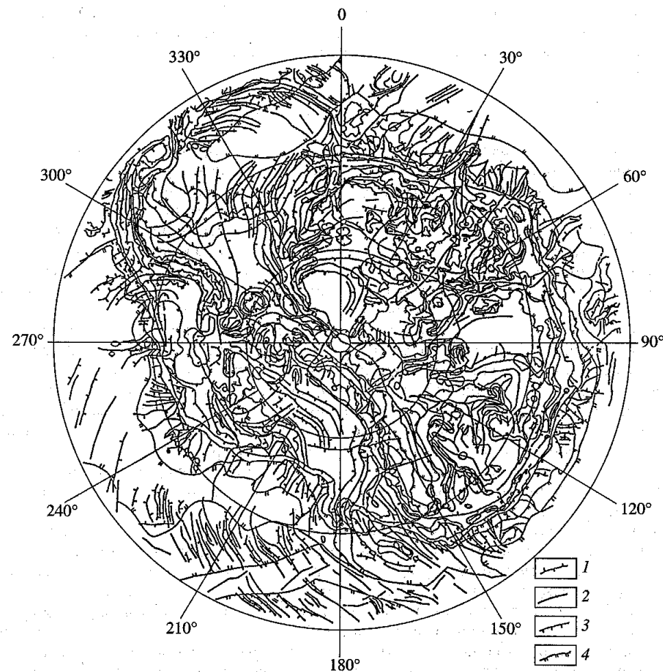
Рис. 1. Карта структурных линий в подводно-подледном рельефе Антарктики Структурные линии: 1 – гребневые, 2 – килевые, 3 – выпуклых перегибов, 4 – вогнутых перегибов
