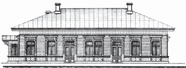
Пассажирское здание станции 4 класса Бологое-Псковской ж/д виды с платформы, с подъезда, в разрезе
