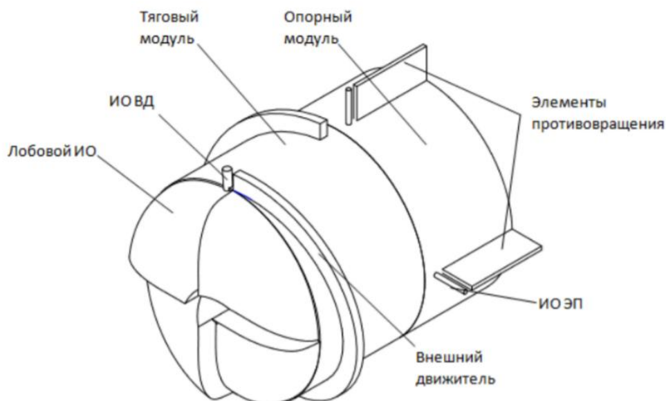
Рисунок 1. Общий вид проходческого подземного аппарата класса Геоход
