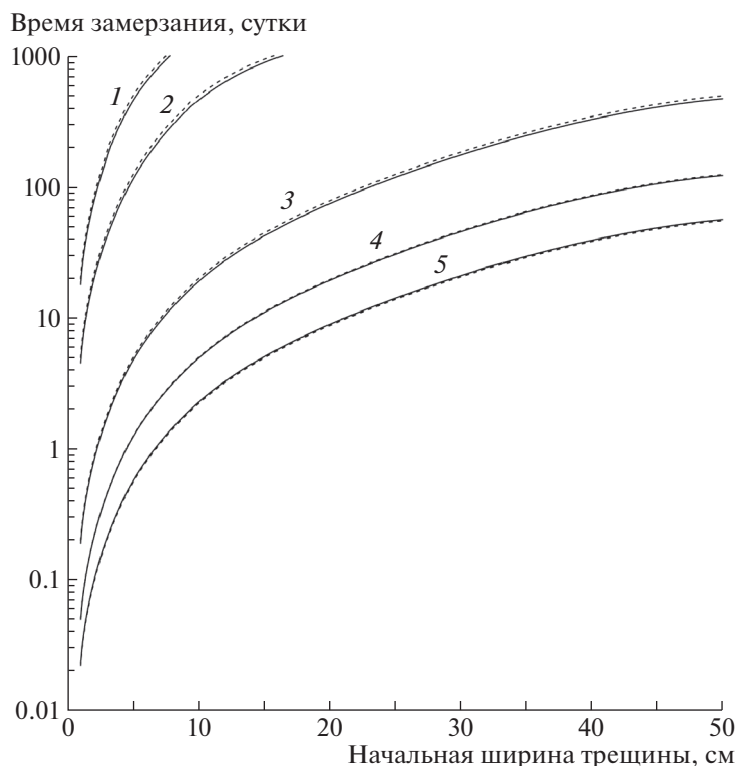
Рис. 5. Время заморозки воды в трещине при различной ширине и температуре ледяной толщи: температура льда: -0.5^{\circ}\text{C} (1); -1.0^{\circ}\text{C} (2); -5.0^{\circ}\text{C} (3); -10.0^{\circ}\text{C} (4); -15.0^{\circ}\text{C} (5). Утолщенной линией показаны значения, полученные в рамках представленной модели, а пунктирной — результаты расчетов по соотношению (16).
