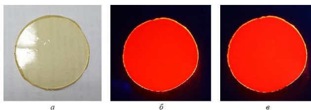
Рис. 1 – Пленка на основе полисилоксан(пропиленоксид)мочевинуретановой матрицы, допированной ионами \text{Eu}^{\text{III}} и кремнийорганическим лигандом при дневном свете (а), при облучении светом \lambda=254 нм (б), при облучении светом \lambda=365 нм (в).
