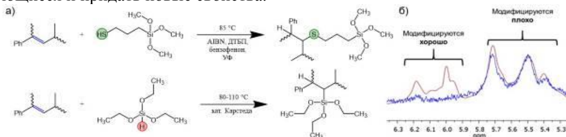
Рис. 1 - а) Реакции гидротииолирования и гидросилилирования смолы С9; б) наложенные сигналы двойных связей исходной смолы и модифицированной.
