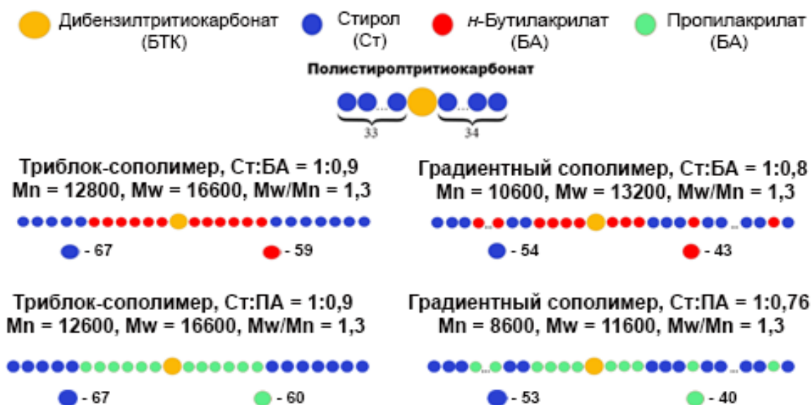
Рис. 1 - Микроструктура стирол-акриловых сополимеров.
