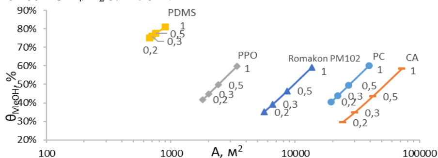
Рис. 1. – Зависимость требуемой площади мембраны (A) и степени извлечения метанола ( \theta_{\text{MeOH}} ) от типа мембраны и давления пермеата (0,2-1,0 атм) при достижении ТТРв -20 °С.
