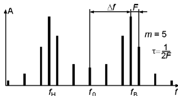
Рисунок 6 – Спектр ЧМн.
