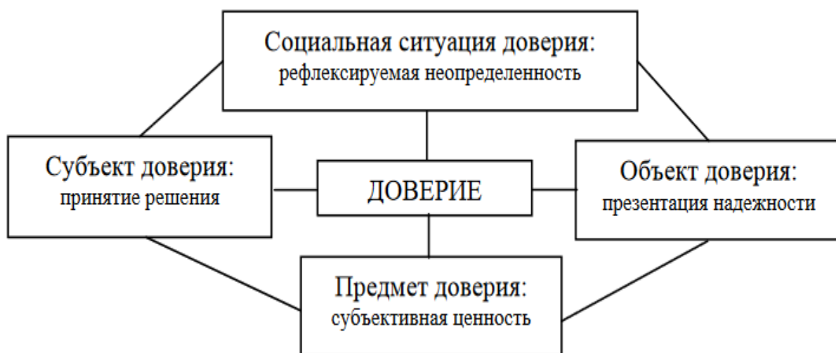
Рис. 3. Структура доверия
