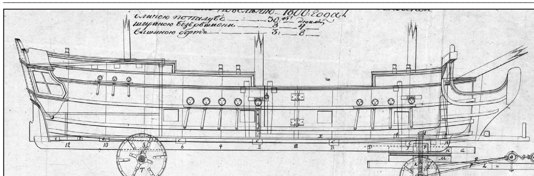
Ил. 3. П. Попов. «Чертёж...». Фрагмент: вид сбоку (изображение повёрнуто в горизонтальное положение)
