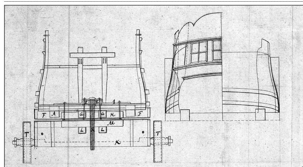
Ил. 4. П. Попов. «Чертёж...» Фрагмент: сечение и вид сзади
