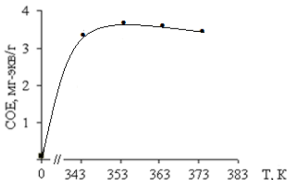
Рис. Зависимость СОЕ по NaOH полимерного комплексона полученных гидролизом СМА-1 сорбентов от температуры реакции.
