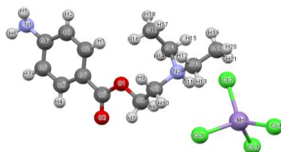
1-rasm. Olingan 2(C_{13}H_{21}N_2O_2), Cl_4 Mn li kompleks birikmaning tasviri. Mnli-kompleks birikmaning kristallografik ma‘lumotlari va strukturasiga aniqlik kirituvchi parametrlar.
