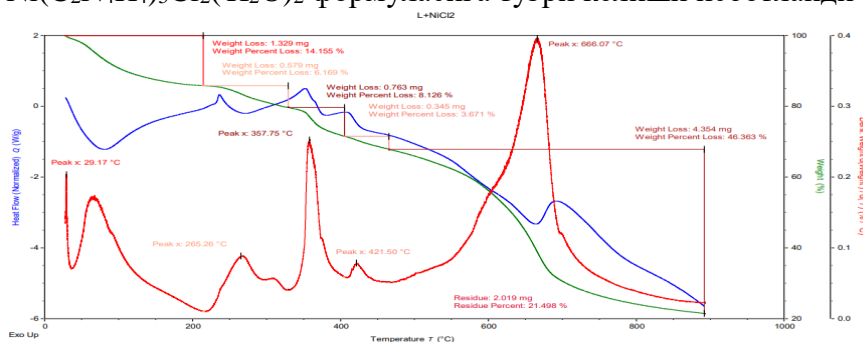
2 – расм: [NiL_5]Cl_2(H_2O)_2 комплекс бирикмасининг термограммаси
