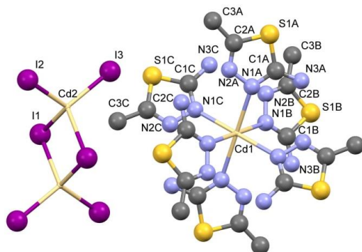
1-расм. Гексакис(2-амино-5-метил-1,3,4-тиадиазол-N) кадмий(II) гексакис(бис-μ-йодо)тетрайодо-дикадмий(II) комплексининг кристалл тузилиши.
