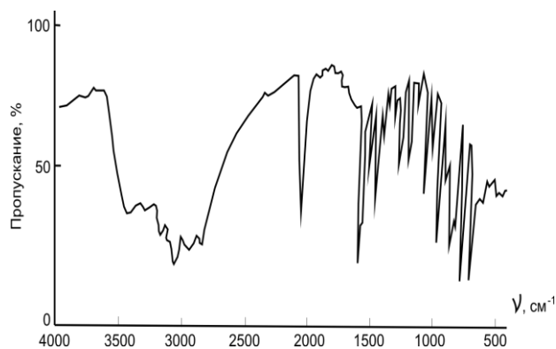
Рисунок 4. ИК-спектры поглощения молекулы [MoO₂(СКБА)·Н]₂·Сl₂.
