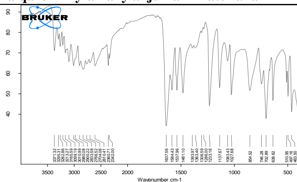
1.rasm. 3-amino-5-merkapto-1,2,4-triazolning IQ spektri
