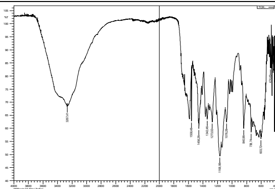
2-rasm. Para-[bis-1,4-(4,4,4-triflorbutandion-1,3)]-benzol tiosemikarbazoni molekulasi ning IQ spektri
