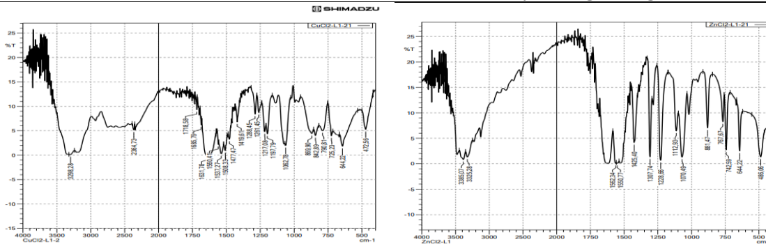
1 (a,b) – rasm: 3-amino 1,2,4-triazol ligandning mis va rux (II) –xloridlar bilan hosil qilgan kompleks birikmalarining IQ-spektroskopiyasi
