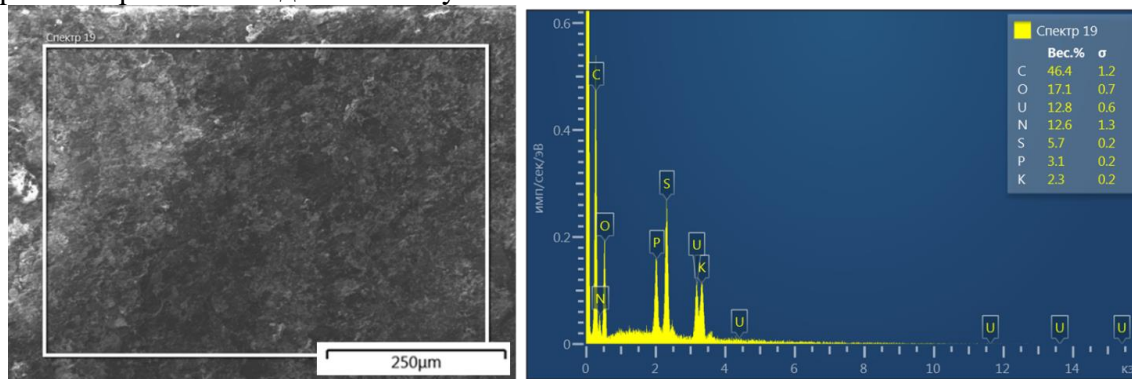
1-расм. [\text{UO}_2(\text{L}^1)_2(\text{L}^2)] комплекс бирикмасининг микроструктураси ва СЭМ-ЭДС элемент анализи
