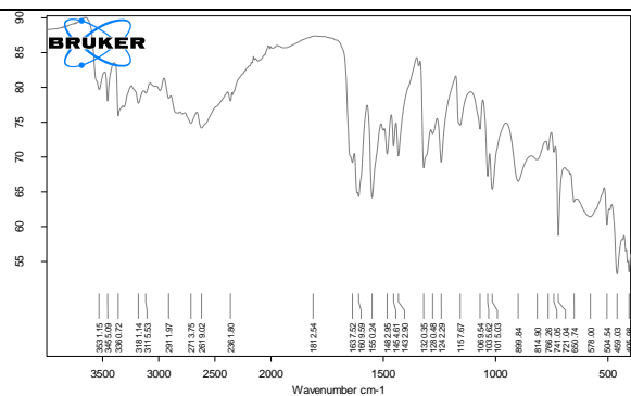
2.rasm. 3-amino-5-merkapto-1,2,4-triazol bilan CdJ 2 tuzi bilan kompleks birikmasining IQ spektri
