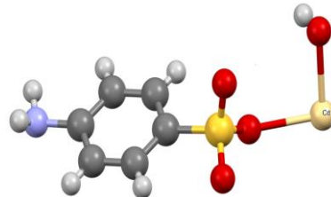
Рис.2. Полимерный комплекса [Cd(H_2O)_2](H_2NC_6H_4SO_3)_2 .
