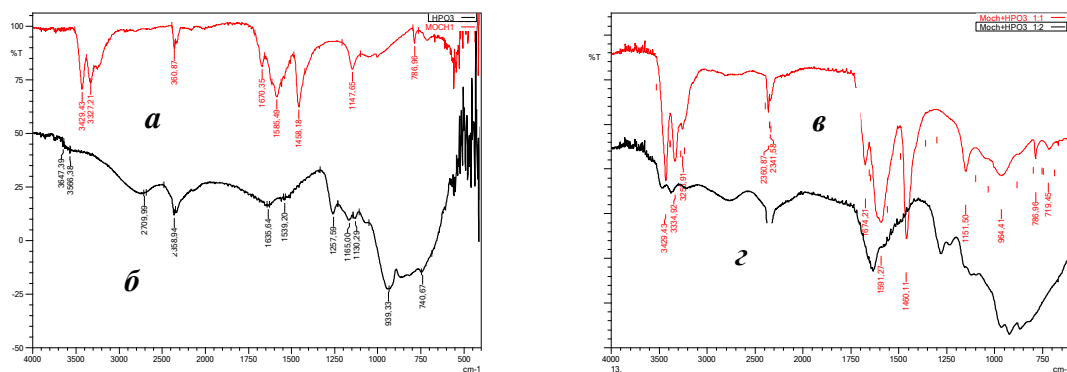
Рис1 ИК-спектры: а- мочевина; б- метафосфорной кислоты в – [\text{CO}(\text{NH}_2)_2 \cdot \text{HPO}_3] ; г- [\text{CO}(\text{NH}_2)_2 \cdot 2\text{HPO}_3]
