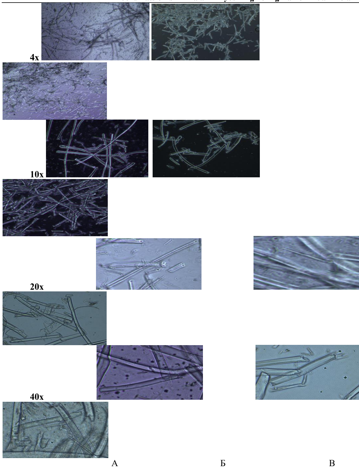
Рисунок. Микроскопические снимки продуктов гидролиза кокона тутового шелкопряда раствором NaOH при концентрации – 0,63 н., времени гидролиза 90 минут, при увеличении в 4, 10, 20, 40 при температурах: А – 323 К; Б – 343 К; В – 373 К.
