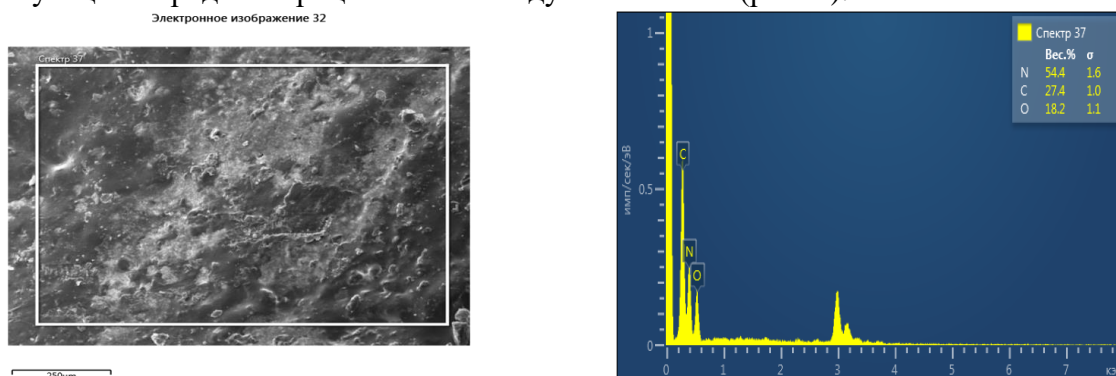
Рис. 2. Изображение в СЭМ и элементного анализа комплексообразующего сорбента КФ-ДТ
