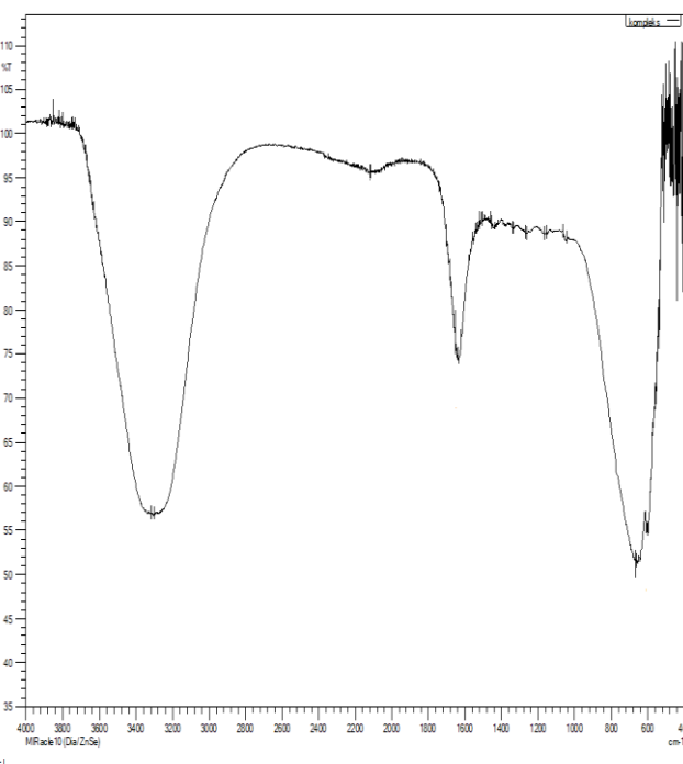
Рис.12. ИК-спектр комплекса меди (II) с 2,7-динитрозо-1,8-диоксинафталин-3,6-дисульфокислоты
