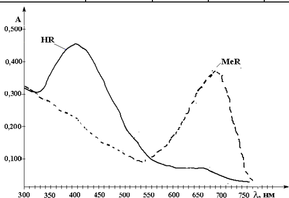
Расм 1. Темир(III) нинг 6-сульфо-1-нитроза-2-нафтол реагенти билан ҳосил қилган комплексининг ютилиш спектри
