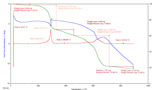
4 – rasm: [CuL_5]Cl_2 kompleks birikmasining termogrammasi
