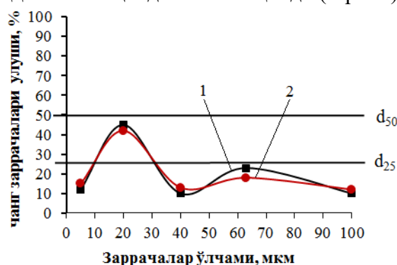
3-расм. Суперфосфат чангининг дисперс таркибини таққослаш графиги 1 – элак анализи; 2-микроскопик анализ
