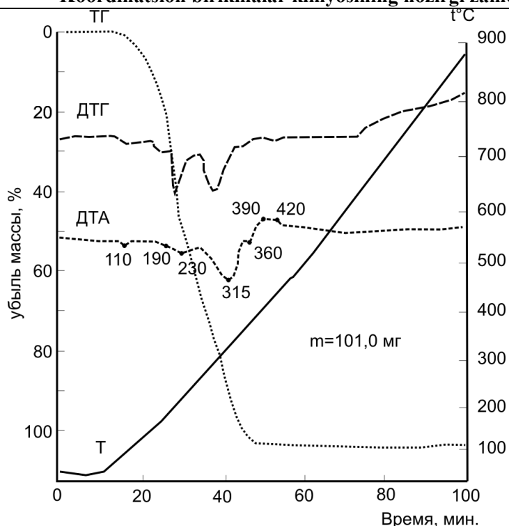
Рисунок 5. Дериватограмма свободного молекулы SKnOBA.
