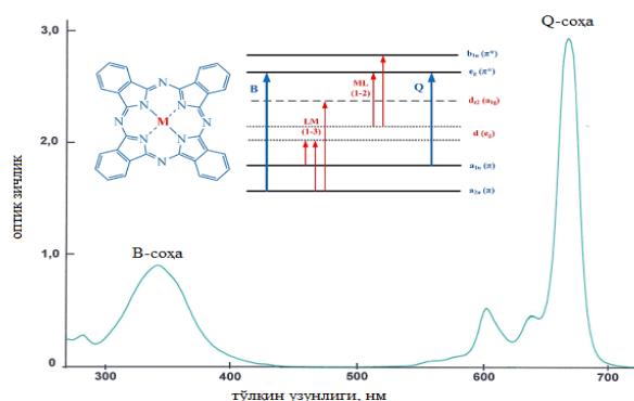
1-расм. МРс нинг электрон ютилиш спектри (тетрагидрофурандаги ZnPc эритмаси мисолида), шунингдек МРс учун зарядланган молекула ўтказишининг умумий схемаси [3; 6800-6806 б.].
