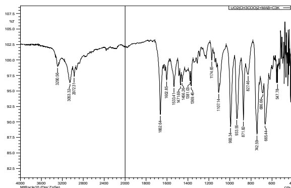
2-расм. [\text{UO}_2(\text{L}^1)_2(\text{L}^2)] комплекс бирикманинг ИҚ-спектри
