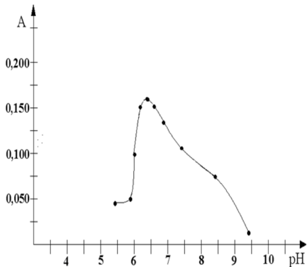
Расм 1. Комплекс бирикма оптик зичлигининг муҳит кислоталилигига боғлиқлиги графиги
