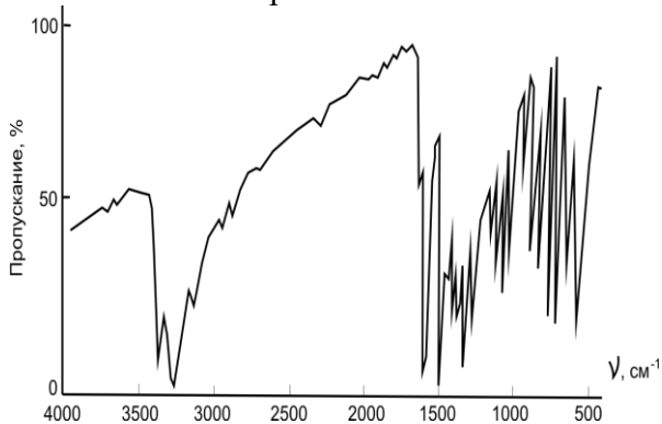
Рисунок 3. ИК-спектры поглощения молекулы семикарбазона бенальдегида.
