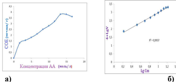
Рис. Зависимость СOЕ синтезированного поликомплексона от концентрации АА (а) и скорости превращения от концентрации АА в логарифмических координатах (б) (Т = 403К; t = 300 мин)
