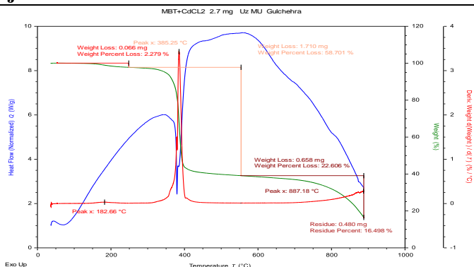
1-Расм. [Cd(C_7H_4NS_2)_2] комплекс бирикманинг дериватограммаси
