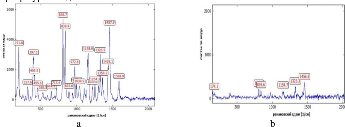
2-расм. 2,4-дихлорфеноксисирка кислотасининг аморф ҳолати(а) ва сувли эритмаси (б) 0-2000 \text{cm}^{-1} ораликда олинган Раман-спектри
