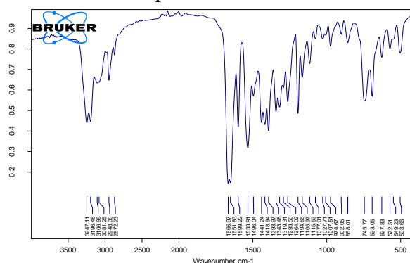
1-rasm. N-fenil-3-oksobutanamid malon kislotaga digidrazidi IQ – spektri
