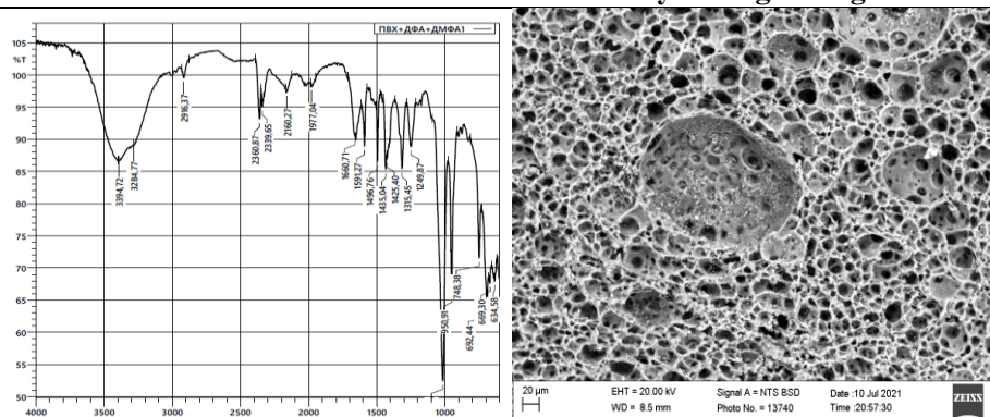
2-расм. Синтез қилинган сорбентнинг ИҚ спектрилинган сорбентларининг микроструктураси
