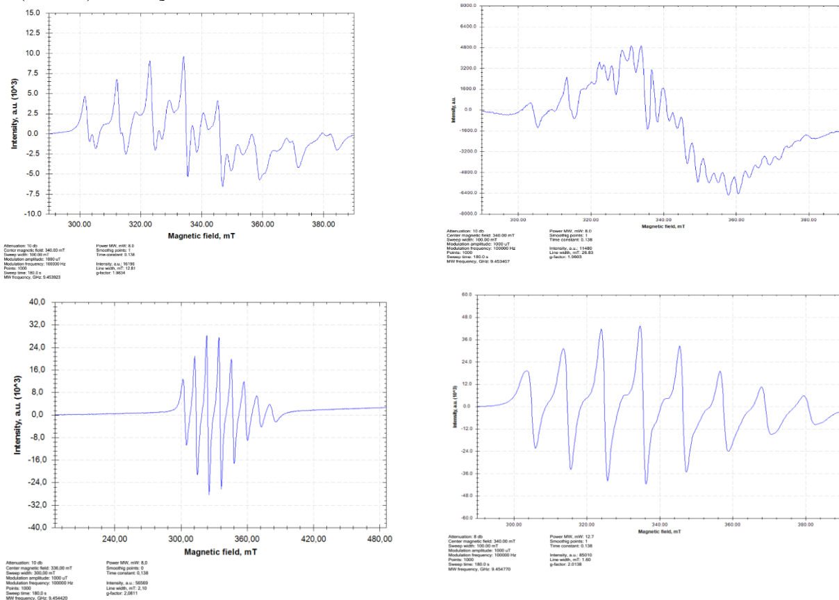
Рис.1.ЭПР спектры синтезированного комплекса [\text{VO}(\text{CF}_3\text{COO})_2 \cdot 3\text{H}_2\text{O}] по реакции (1): а – в метаноле; б - в ацетоне; в - по реакции (1) без этанола; г - по реакции (1) без ЦК.
