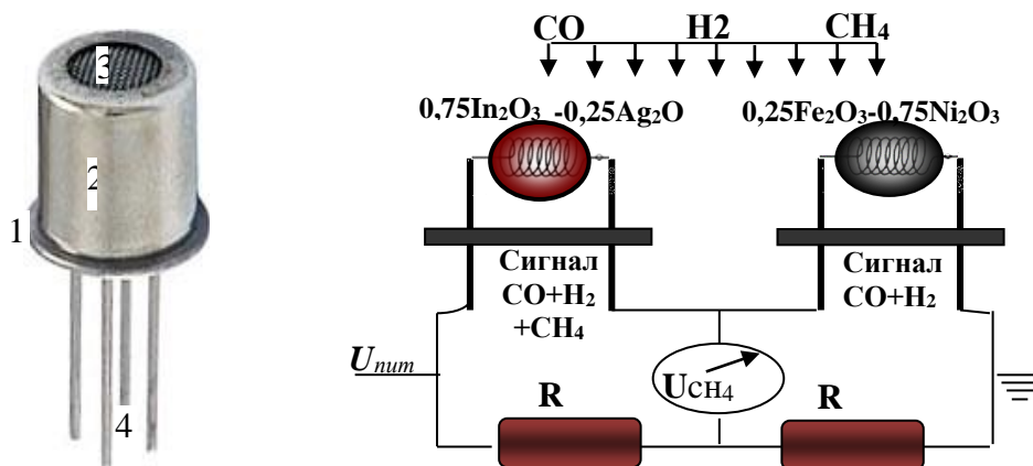
2-расм. Метанни селектив термокаталитик сенсорининг фотосуръати ва схемаси. 1-корпус, 2- химоя қопқоғи, 3-тешикли титан қоплама, 4-металл симлар.
