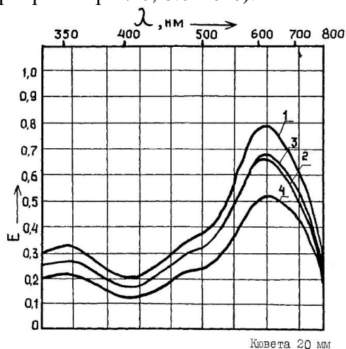
Рис.2. Спектры поглощения йод – крахмальных комплексов: 1, 2, 3 – окисленные с NaClO (соответственно при pH раствора 7.0, 8.0 и 9.0) ( C_{\text{крахмал}}=35\% , C(NaClO)=0,01\% к массе сухого крахмала) и 4 – нативный крахмал ( C_{\text{крахмал}}=35\% .)
