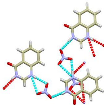
2- rasm. Qatlamlar orasidagi vodorod bog`larning ko`rinishi
