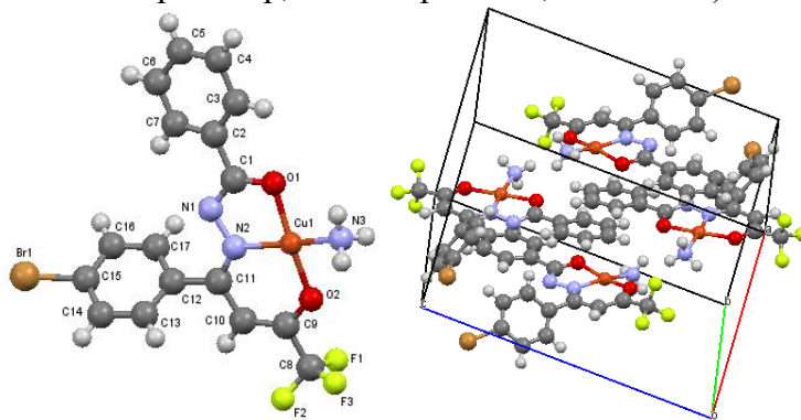
Рисунок 2. Молекулярная структура и упаковки молекул \text{CuL}^5 \cdot \text{NH}_3 .
