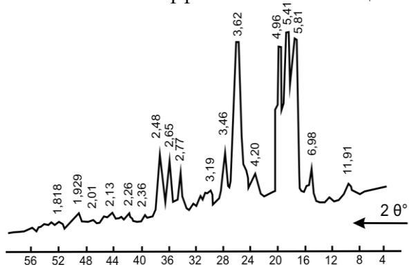
Рисунок 1. Рентгенограмма молекулы семикарбазона параоксибензоальдегид.
