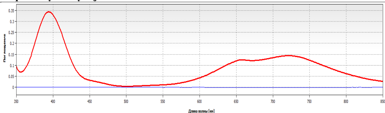
3-rasm. 5-sulfosalitsilning \text{Cu}^{2+} va \text{Ni}^{2+} metallari bilan hosil qilgan koordinatsion birikmalari UB spektrlari.
