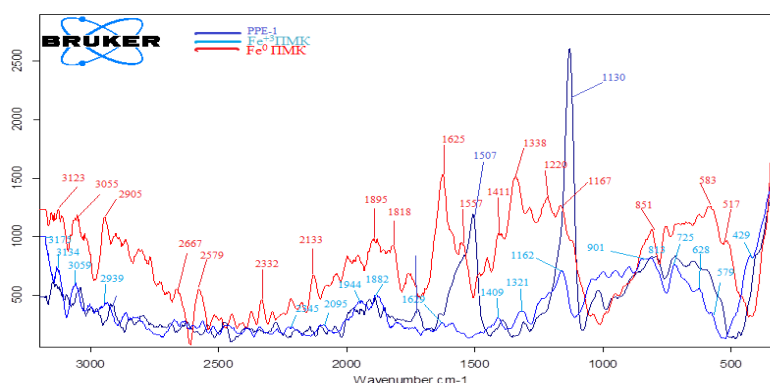
1-рис. Раман спектроскопия комплекса железо-полимер на основе PPE-1 и иона металла Fe(III)
