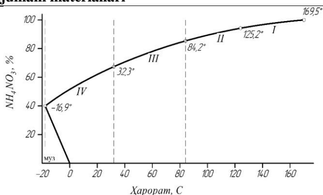
1-расм. \text{NH}_4\text{NO}_3 нинг сувда эрувчанлиги.
