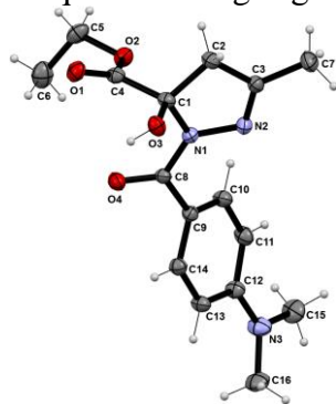
1-rasm. 2,4-dioksopentan kislota etil efir 4-dimetilaminobenzoil gidrazoni molekulyar tuzilishi
