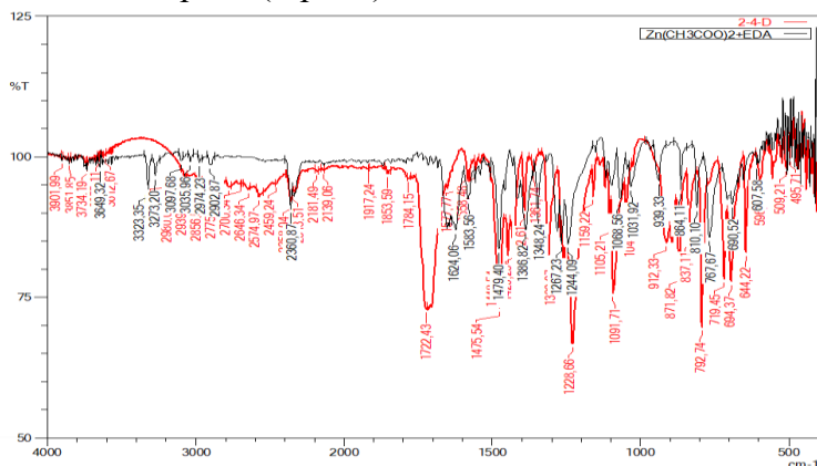
1-расм. [\text{Zn}(2,4\text{-D})_2\text{En}] таркибли комплекс бирикма ИҚ-спектри.
