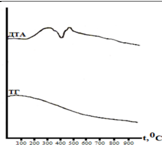
Рис.2 Дериватограмма фосфорнокислого катионита
