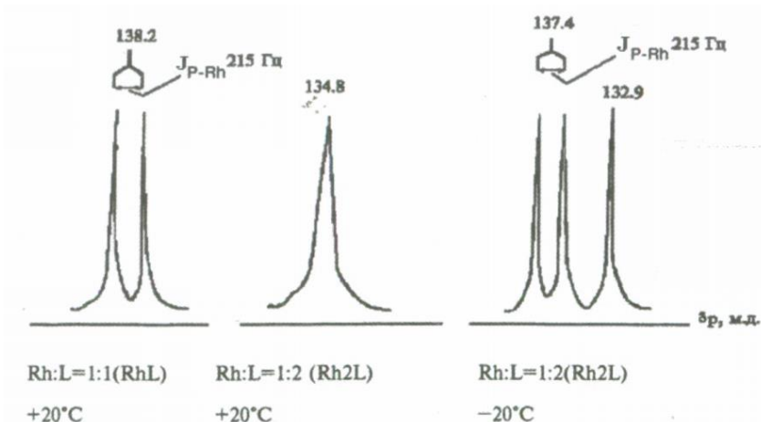
Рис.2. Зависимость характера спектров ЯМР 31 P координационных систем RhL и Rh2L от соотношения M:L и температуры
