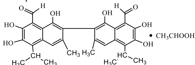
2-расм. Госсипол сирка кислотасини структура формуласи.
