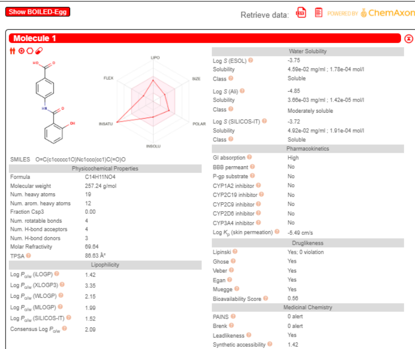
Рис.1. Вычисленные значения параметров сгруппированы в различных разделах однопанельной молекулы (физико-химические свойства, липофильность, фармакокинетика, сходство с лекарственным средством и лекарственная химия).
