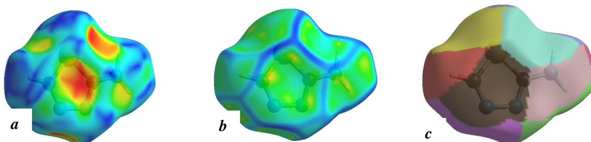
2-расм. 2-амино-1,3,4-тиадиазол a -шакл қўрсаткичлари майдони, b -ўзаро таъсир худудларини қўрсатадиган эгри чизиқ майдони ва қисмларга бўлиниш майдони тасвири
