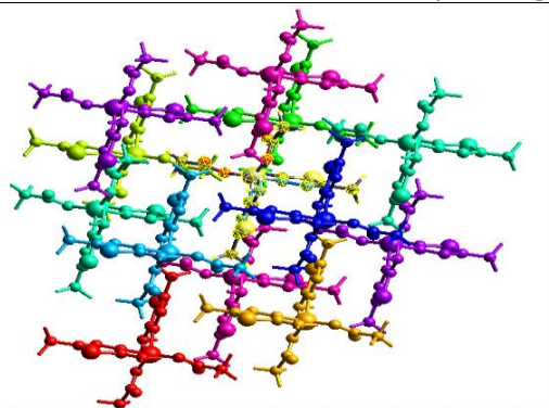
4-расм. Танланган (сарик нур) молекула атрофидаги молекулалар турли хил рангларда кўрсатилган.
