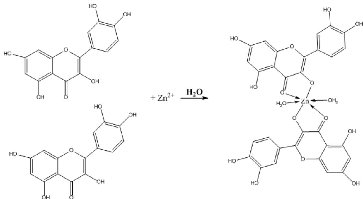
1-rasm. Kversetinning Zn(II) kationi bilan kompleks hosil qilish sxemasi
