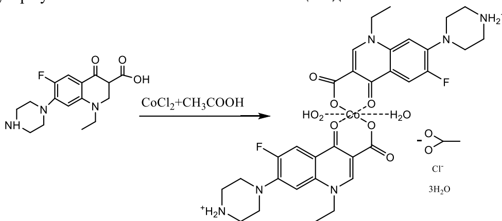
1-расм. [Co(HL)_2(H_2O)_2](CH_3COO)Cl(H_2O)_3 таркибли комплекс бирикма синтези реакцияси.
