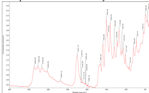
Рис.1. ИК-спектр ионита на основе ДГК+ФК
