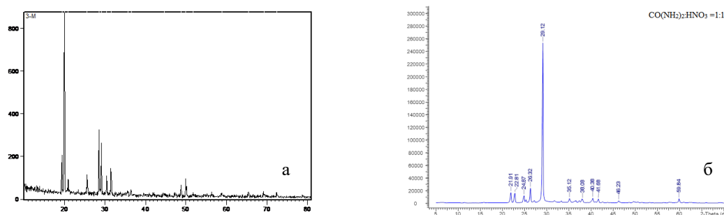
Рис. 1. Дифрактограмма: а) мочевины б) мононитромочевины
