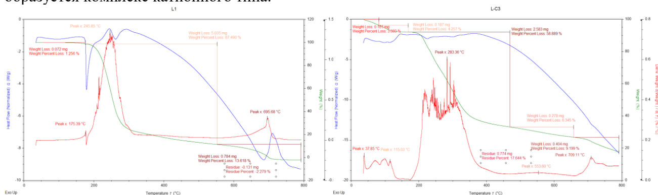
Рис. 2. Термограмма лиганда L (А) и комплексного соединения [CuL 4 Br]Br(Б)
