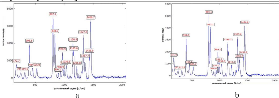
3-расм. [Zn(2,4-D) 2 En] таркибли комплекс бирикмасининг кристалл ҳолатида (а) ва сувли эритмаси (б) 0-2000 см -1 оралиқда олинган Раман-спектри
