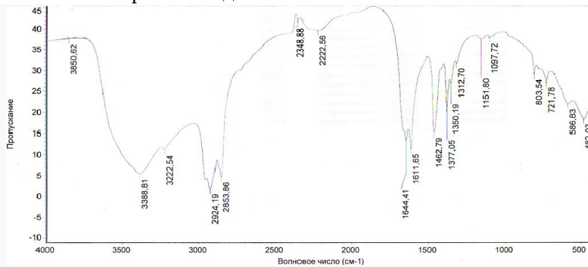
Рис. 1. ИК-спектр комплекса Fe(III)-L 2 .
