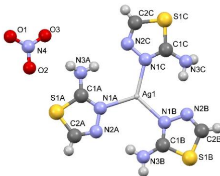
1-расм. Трис(2-амино-1,3,4-тиадиазол-N) кумуш(I) нитрат комплексининг кристалл тузилиши.
