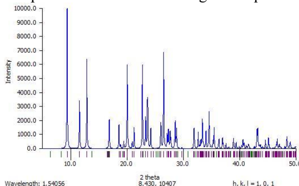
2-rasm. Polimer kompleks birikmaning diffroktogrammasi
