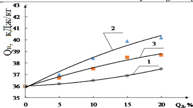
1-rasm. Olingan ko‘mir briketlarining birlashtiruvchi moddalar miqdoriga qarab kalorifik qiymatining o‘zgarishi: natriy silikatning 1-5% suvdagi eritmasi; 2-gossipol smolasi; 3 - piva bardasi
