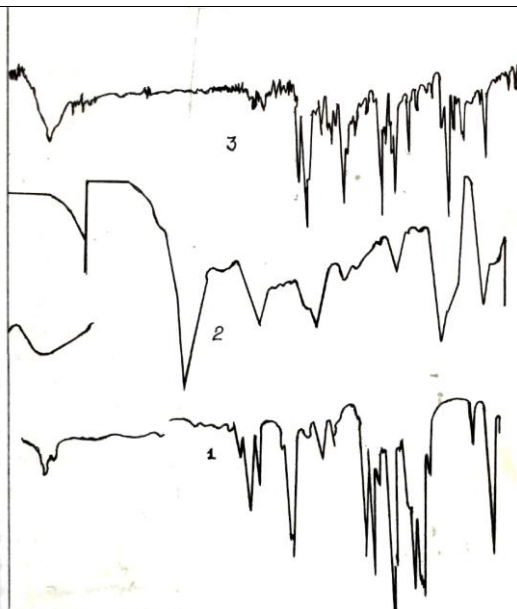
Расм 1. Эпихлоргидин (1) эпихлоргидин билан бензоксазолтион асосида олинган олигомер (2), шу олгомерни Ni^{+2} билан комплекси(3) ИҚ-спектрлари
