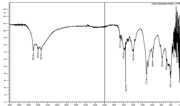
3-rasm. Para-[bis-1,4-(4,4,4-triflorbutandion-1,3)]-benzol tiosemikarbazoni Zn(II) kompleks birikmasining IQ spektri
