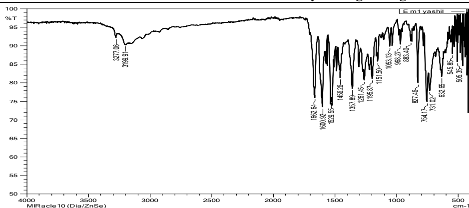
1-rasm. Asparagin kislota aroilgidrazonining Cu(II) ion bilan hosil qilgan komrleks birikmasi IQ spektri.
