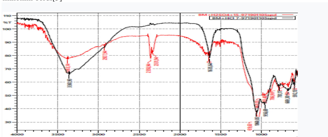
3-rasm. Vermikulitga 15%li sulfat kislota va 7%li xlorid kislotalarda aktivlantirib olingan moddalarning IQ tahlili.(bunda qizil chiziqlar 15%li sulfat kislota va qora chiziqlar 7%li xlorid kislotaning egri chiziqlari.)
