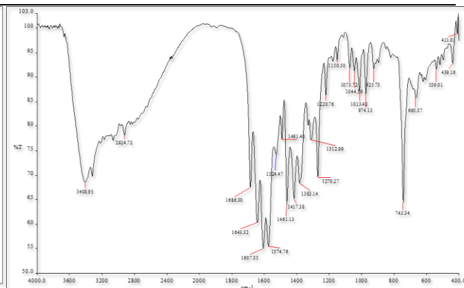
2-расм. [\text{CoL}_2(\text{SO}_4)_2] \cdot \text{H}_2\text{O} комплексининг ИҚ-спектри
