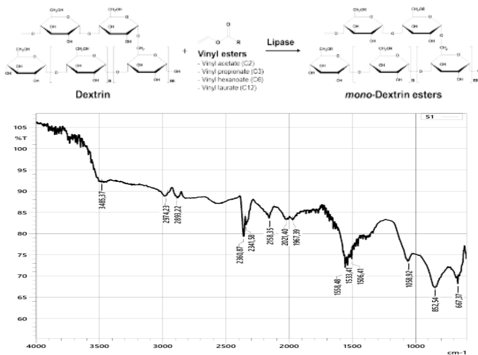
1-Rasm. Sintez qilingan dekstrinni IQ spektri
