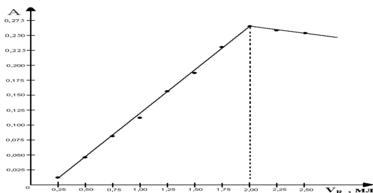
Расм 1. Комплекс бирикма оптик зичлигининг қўшилган реагент миқдорига боғлиқлиги графиги
