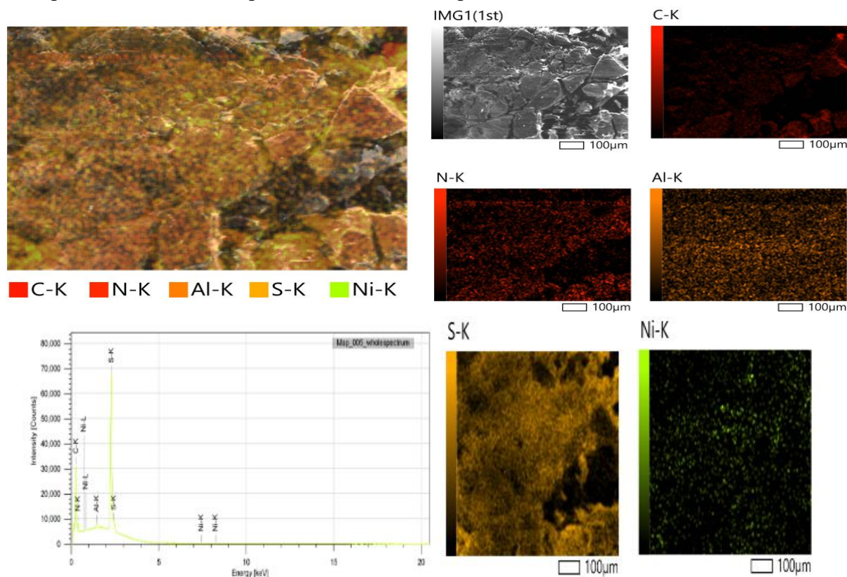
Рис.2. Микроструктура комплексного соединения [NiL_1] и данные ЭДА
