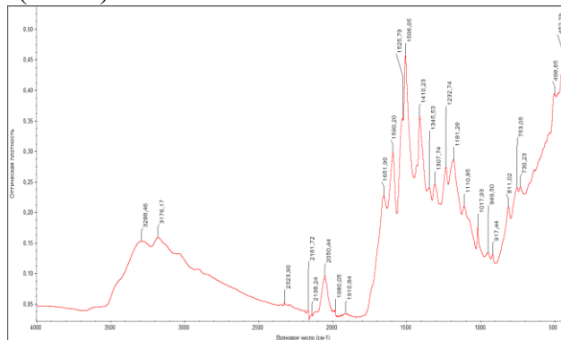
Рис.2. ИК спектр иона Cu(II), поглощенного ионитом ДГК+ФК
