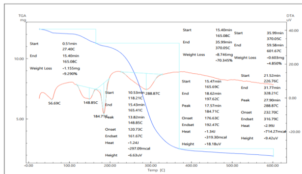
2-расм. [Gd(2\text{-МВТ})_3] термограммаси
