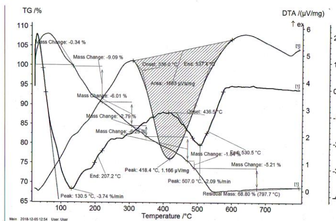
Рис. 2. Кривые термического анализа комплекса Fe(III)-L 2 .
