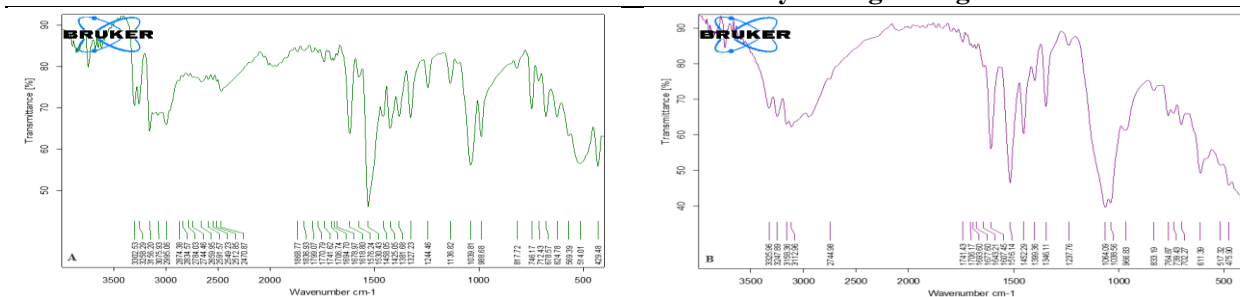
Рис. 1. ИК–спектр лиганда (А) и комплекса (Б) на его основе
