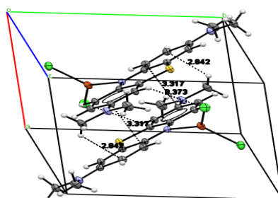
5-rasm. [Mk]CuCl 2 uchun qisqa masofalar diagrammasi.
