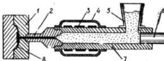
1-rasm. Bosim ostida quyish sxemasi: 1 - qarshi qolipi; 2 - ko'krak; 3 - elektr isitgichlar; 4 - korpus; 5 - bunker; 6 - piston; 7 - qabul qiluvchi kamera; 8 - detal.
