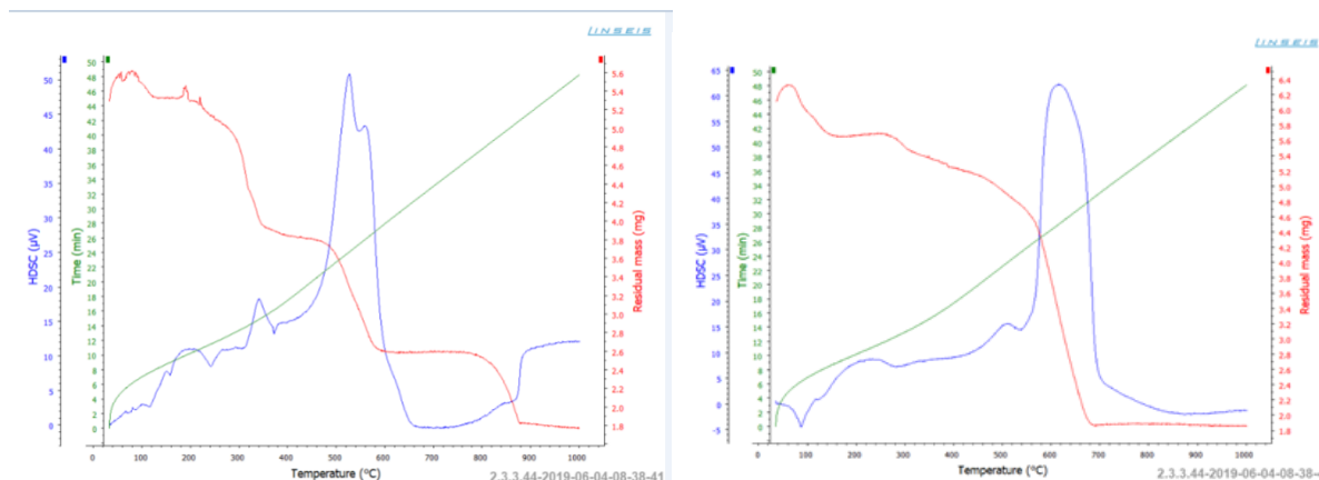
3.23-расм. [MnL 2 (NO 3 ) 2 ] \cdot 2H 2 O ва [ZnL 2 (NO 3 ) 2 ] \cdot 2H 2 O комплексининг дериватограммаси
