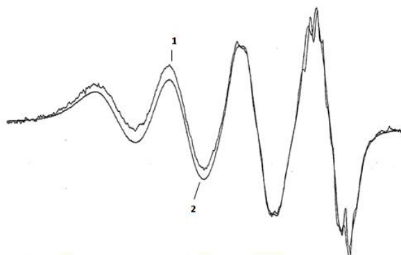
Рисунок 1. Спектр ЭПР комплексного соединения CuL^1 \cdot NH_3 в растворе толуола при комнатной температуре: 1- экспериментальный спектр, 2- теоретически построенный спектр.
