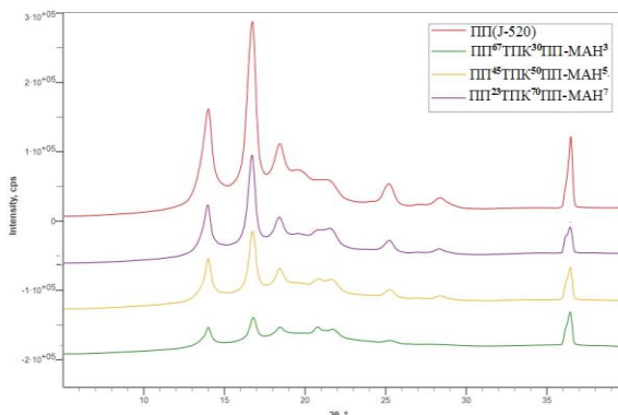
1-расм. Композицион материалларнинг рентген диффрактограммалари Композиция намуналарида ТПК миқдори ортиб бориши билан уларнинг механик хусусиятлари пасайиб бориши кузатилди.
