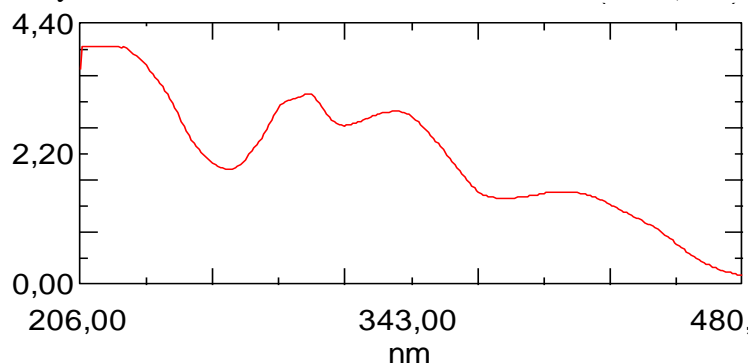
2-rasm. Asparagin kislota digidrazidining Cu(II) ion bilan hosil qilgan kompleks birikmasining etanoldagi 0.001% li eritmasidan 200-900 nm oralig'ida olingan UB spektri.
