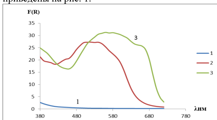
Рис.1. Спектры отражения сорбента ППА-1(1), реагента фенилфлуорона (2), и его комплекса с ионами молибдена (3).
