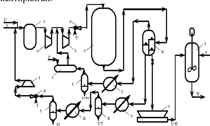
Расм 1. Юқори босимда этиленнинг гетероҳалқали метакрилат билан сополимерлари ва улар асосидаги қўндирмалар олиниш технологик схемаси 1 – резервуар; 2, 3 –компрессорлар; 4 – инъекцион аралаштиргич; 5– қувурли реактор; 6, 8, 10, 13 – ажратгичлар; 7, 9, 14 – совутгичлар; 11 – компрессор; 12 – мономер идиши; 15 – экструдер; 16 – аралаштиргич.
