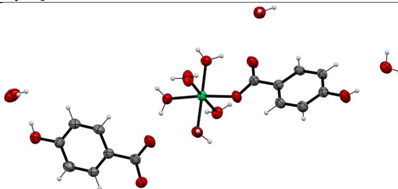
1- расм [Ni(4\text{-ГБК})(H_2O)_5](4\text{-ГБК})(H_2O)_3 молекуласининг тузилиши.
