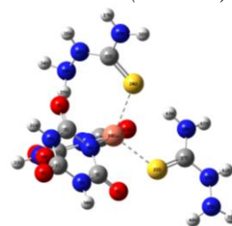
4-rasm. Cu(II) kompleksining fazoviy tuzilishi
