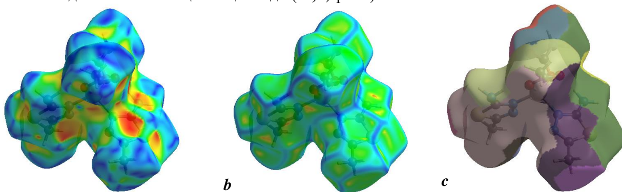
2-расм. Бис(2-амино-5-метил-1,3,4-тиадиазол-N) диацетато рух(II)нинг a -шакл кўрсаткичлари майдони, b -ўзаро таъсир ҳудудларини кўрсатадиган эгри чизик майдони ва c -қисмларга бўлиниш майдони тасвири
