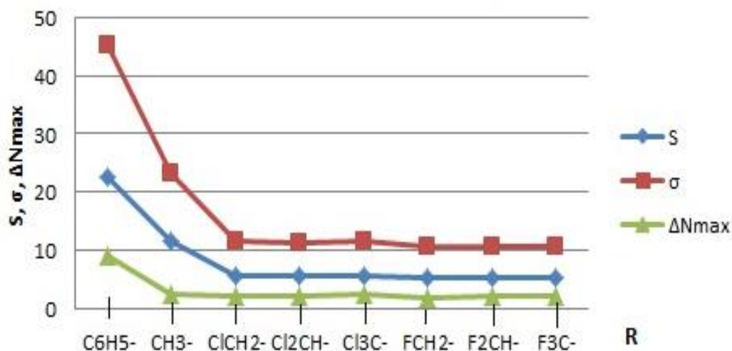
2-grafik. [VO(RCOO) 2 ·Solv] tarkibli kompleksdagi R tarkibining KKH yordamida aniqlangan σ, S, ΔN max parametrlari bog'liqlik grafigi
