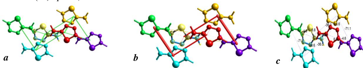
3-расм. 2-амино-1,3,4-тиадиазол танланган молекуласининг ва бошқа рангли молекулалар орасидаги ўзаро таъсир энергиялари: a – дисперсион таъсир, b – электростатик ва c – умумий
