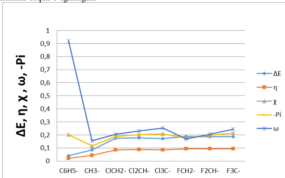
1-grafik. [VO(RCOO) 2 ·Solv] tarkibli kompleksdagi R tarkibining KKH yordamida aniqlangan ΔE, χ, η, Pi, ω, parametrlari bog'liqlik grafigi
