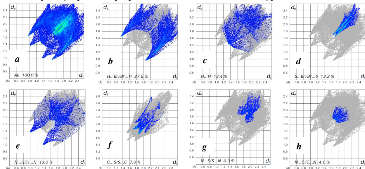
2-расм. Бис(2-амино-1,3,4-тиадиазол-N) дибромид рух(II) молекуласининг икки ўлчовли бармоқ излари майдонлари ва уларнинг Хиршфельд юзасига нисбий ҳиссаси.
