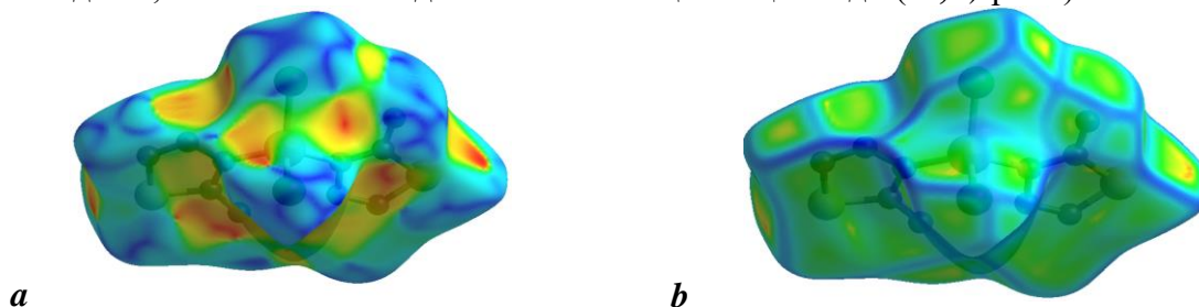
1-расм. бис(2-амино-1,3,4-тиадиазол-N) дибромид рух(II) а-шақл кўрсаткичлари майдони ва б-ўзаро таъсир ҳудудларини кўрсатадиган эгри чизиқ майдони
