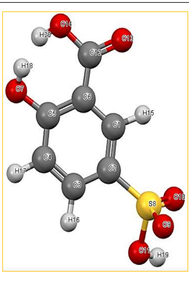
1-rasm. 5-sulfosalitsil kislota ning molekulyar dinamik usul bilan zaryadlar taqsimoti.
