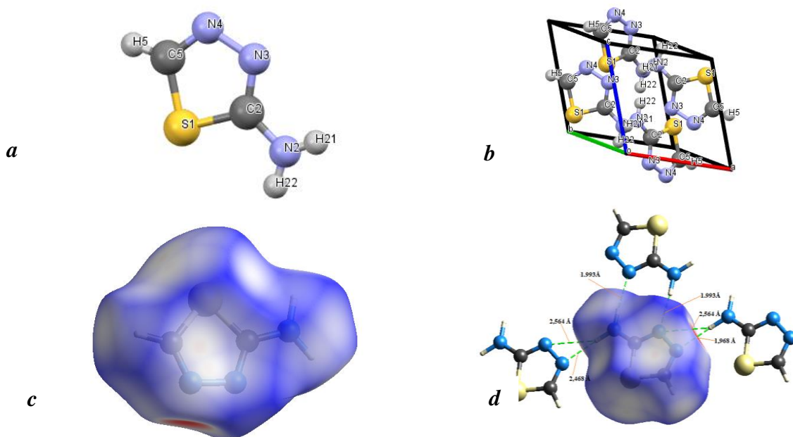
1-расм. 2-амино-1,3,4-тиадиазол a - кристалл тузилиши, b - кристалл таҳлами, c - Хиршфельд юзаси таҳлили, d -молекулалар аро водород боғланиши
