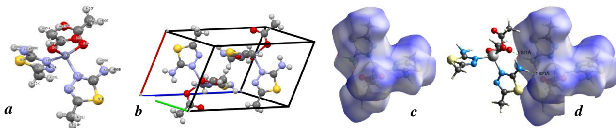
1-расм. Бис(2-амино-5-метил-1,3,4-тиадиазол-N) диацетато рух(II)нинг a - кристалл тузилиши, b - кристалл таҳлими, c -Хиршфельд юзаси таҳлили, d -молекулаларо водород боғланиши
