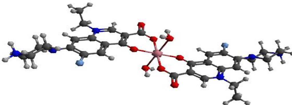
2-расм. [Co(HL) 2 (H 2 O) 2 ](CH 3 COO)Cl(H 2 O) 3 комплексининг kvartet spin-eIektron xolatida maqбуллаштирилган геометрияси.
