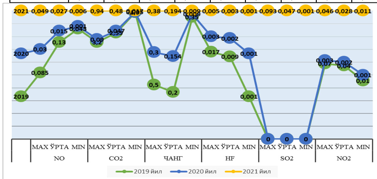
1-расм. Атмосфера ҳавосидаги зарарли моддаларнинг 2019-2021 йиллардаги миграцияси диаграммаси
