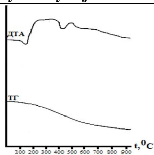
Рис.1 Дериватограмма сульфокатионита
