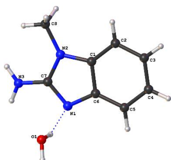
Рис. 1. Геометрическое строение I
