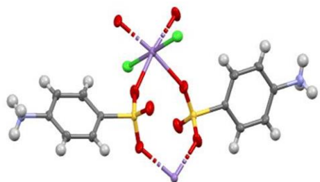
Рис.1. Структура МОП-1
