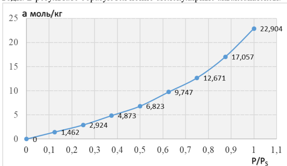
Рис.3. Изотерма адсорбции вода на металлоорганическом полимер MOF-1
