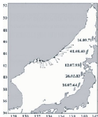
Рис. 2. Величина вертикальных и горизонтальных заплесков цунами 1983 и 1993 гг. на побережье Восточного и Южного Приморья (составлено автором по данным [2, 3, 4, 5])
