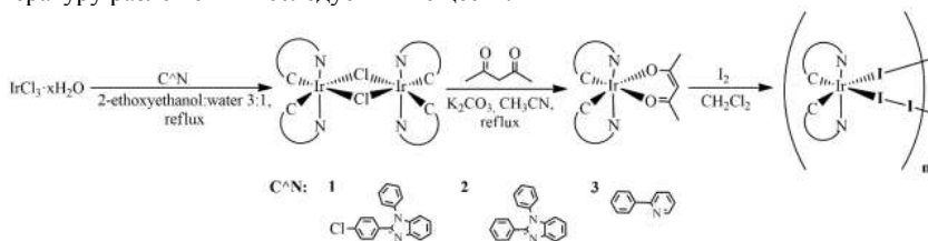
Рис 1. Схема синтеза 1D циклометаллируемых полимеров иридия(III)
