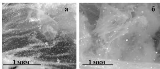
Рис. 1. РЭМ-изображения структур, содержащих частицы \text{CeO}_2 и наночастицы золота полученные а) фотолизом водно-этанольного раствора \text{HAuCl}_4 , б) термолизом целлюлозы, обработанной растворами нитрата церия (III) и тетрахлоороурата (III) водорода.
