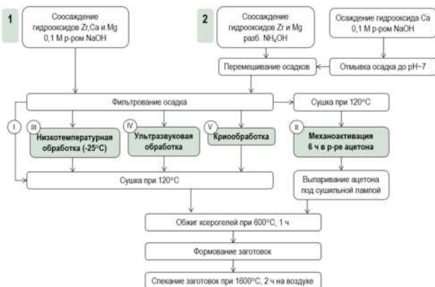
Рис. 1. Схема получения ксерогелей, порошков и керамики в системе ZrO_2 – CaO – MgO
