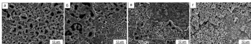
Рис. 1. СЭМ-изображения поверхности ПЭО-покрытий, сформированных на ниобии: а) в 0.1 M \text{Na}_2\text{B}_4\text{O}_7 в течение 10 мин при j_a = 0.1 А/см 2 ; б) в 0.1M \text{Na}_2\text{B}_4\text{O}_7 в течение 5 мин при j_a = 0.1 А/см 2 ; в) в 0.1 M \text{Na}_2\text{WO}_4 + 0.1\text{M} \text{CH}_3\text{COOH} в течение 5 мин при j_a = 0.1 А/см 2 ; г) в 0.1 M \text{Na}_2\text{WO}_4 в течение 5 мин при j_a = 0.2 А/см 2
