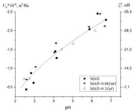
Рис. 1. Электрофоретическая подвижность и электрокинетический потенциал частиц исходных силикатных пористых МАП стекол и композитов МАП+0.08ZnO и МАП+0.5ZnO, содержащих различное количество оксида цинка
