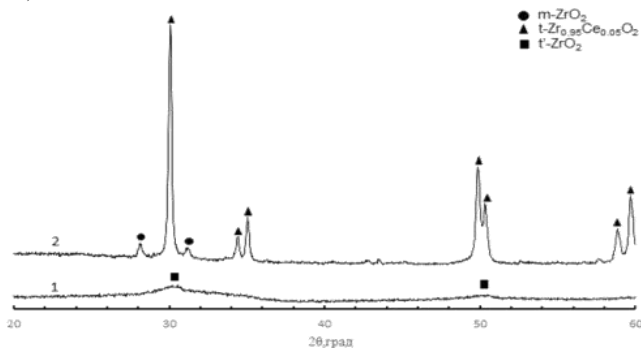
Рис. 1. Дифрактограммы порошка, полученного обжигом механообработанного ксерогеля при 600^\circ\text{C} (1) и керамики, спеченной при 1600^\circ\text{C} (2)
