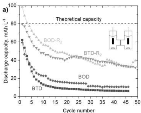
Рис. 2. Зависимость разрядной емкости Н-ячеек от количества циклов
