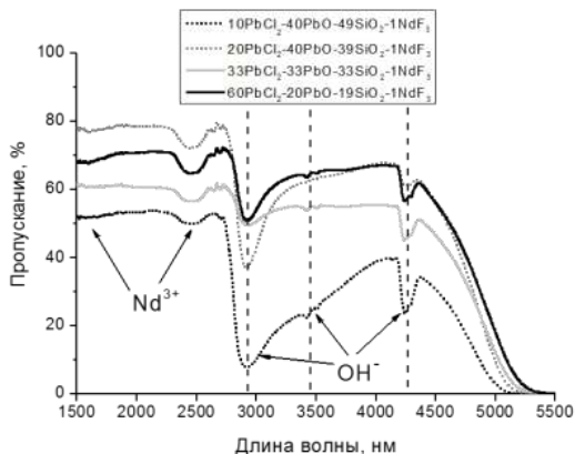
Рис.1. Спектры пропускания стёкол системы \text{PbCl}_2\text{-PbO-SiO}_2 в ИК области
