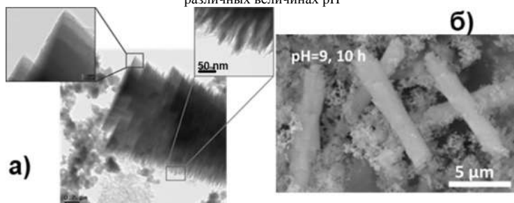
Рис. 2. Изображения ПЭМ (а) и СЭМ (б) образца, полученного при pH 9 и 10 часах изотермической выдержки
