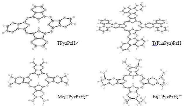
Рис. 1. Молекулярные структуры полученных анионных соединений замещенных тетрапиразинопорфиразинов
