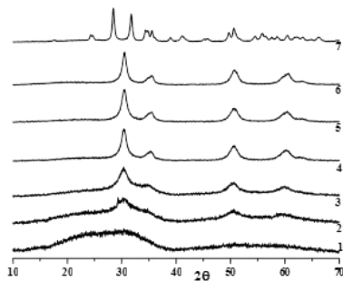
Рис. 3. Рентгеновские дифрактограммы порошков (1-x)\text{ZrSiO}_4-x\text{HfO}_2 , где x = 0.0(1); 0.2(2); 0.3(3); 0.5(4); 0.7(5); 0.8(6); 1.0(7) , после обжига при 850^\circ\text{C} 2 ч.
