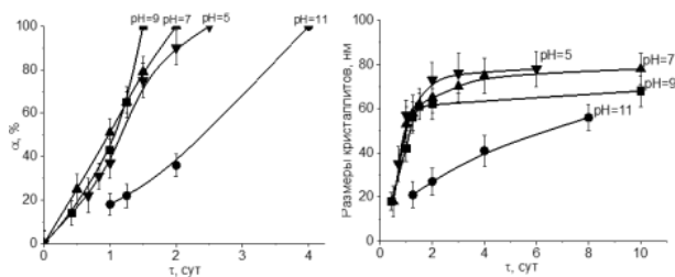
Рис. 1. Зависимость массовой доли фазы ( \alpha ) соединения \text{BiAl}_3(\text{PO}_4)_2(\text{OH})_6 и размеров кристаллитов от продолжительности изотермической выдержки ( \tau ) в гидротермальных условиях при различных величинах pH
