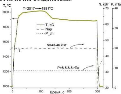
Рис. 1. Изменение температуры поверхности (Т), мощности анодного питания (N) и давления в камере плазмотрона (P) ультравысокотемпературного материала Ta_4HfC_5-30 об.% SiC под воздействием сверхзвукового потока азота
