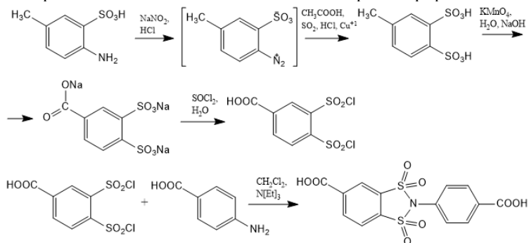
Рис. 1. Синтез 4-карбокси-N-(п-карбоксифенил)-бензол-1,2-дисульфонимида
