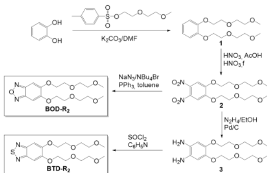
Рис. 1. Синтез BOD-R 2 и BTD-R 2
