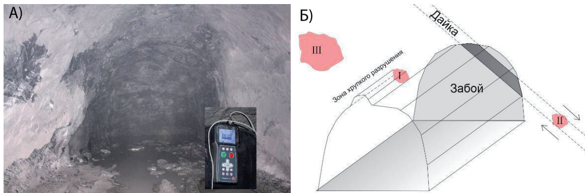
Рис. 3. А) Портативный прибор «Prognoz-L» в горной выработке в проходке. Б) Схематическое изображение трех типов очага неустойчивости, I – процесс динамического заколообразования в кровле или пяте кровли; II – мгновенная подвижка (stick-slip) по дайке или системе трещин; III – очаг, формирующийся в монолитной породе в состоянии объемного сжатия.
