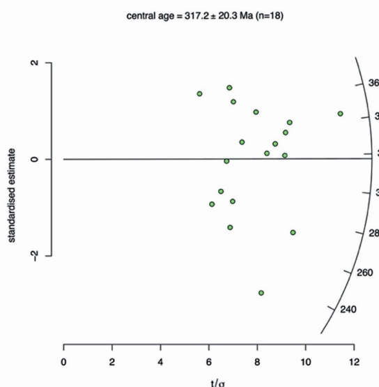
Рис. 2. Радиальная диаграмма распределения трековых возрастов в апатите для образца Repojarvi4 (глубина 9.8 м), полученная с помощью программы IsoplotR (Vermeesch, 2018).
