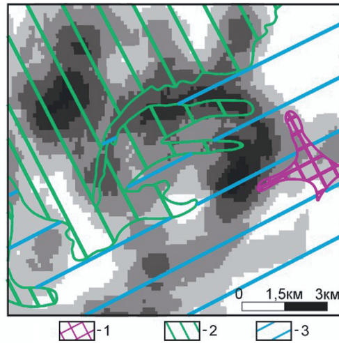
Рис. 4. Северная кольцевидная аномалия: 1 – триас, 2 – мел, 3 – юра. Затемнение – увеличение плотности линеаментов.
