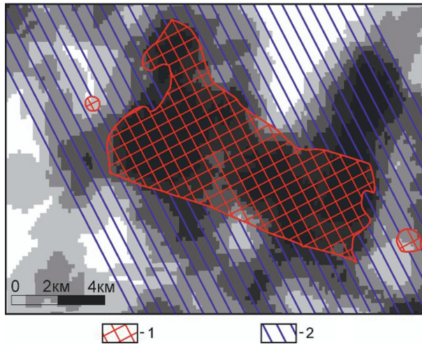
Рис. 3. Аномалия плотности линеаментов в пределах ДКМ: 1 – палеозойский СВК, 2 – мезозойский СВК. Затемнение обозначает увеличение значений плотности линеаментов.
