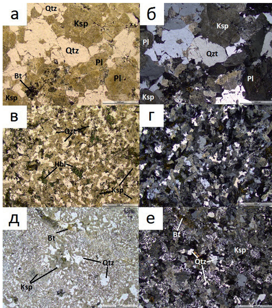
Рис. 1. Петрографические шлифы гранитов: а, б – крупнозернистый биотитовый гранит; в, г – среднезернистый амфиболовый плагиогранит; д, е – среднезернистый гранит с микропегматитовой структурой. а, в, д – изображения шлифов без анализатора, б, г, е – с анализатором.
