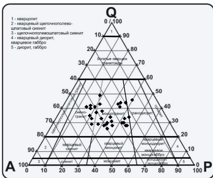
Рис. 2. Диаграмма петрографического состава образцов.
