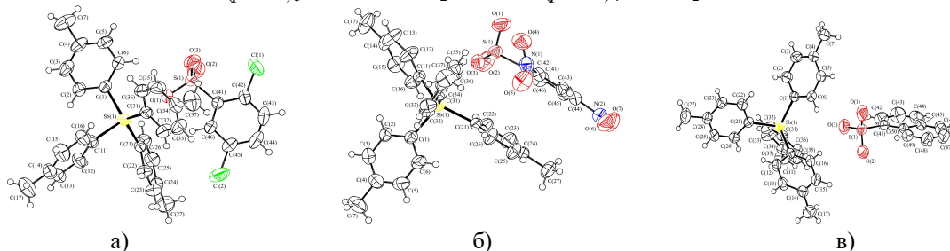
Рис. 1. Структура комплексов аренсульфонатов тетра( пара -толил)сурьмы: а – I , б – II , в – III
