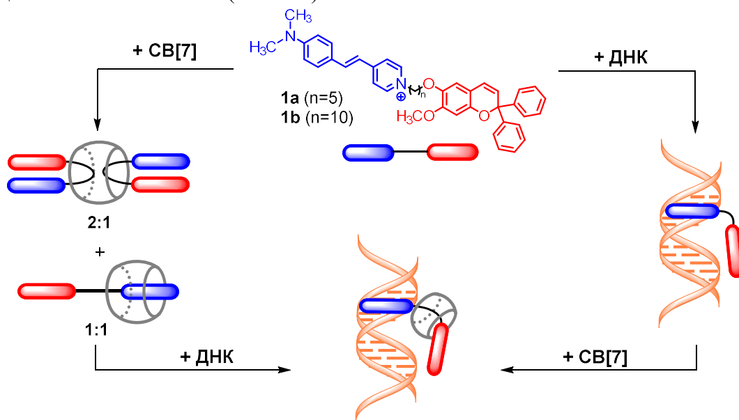
Схема 1. Схематическое представление равновесных процессов, происходящих в растворах двойных и тройных комплексов между конъюгатами 1a-b , ДНК и CB[7].
