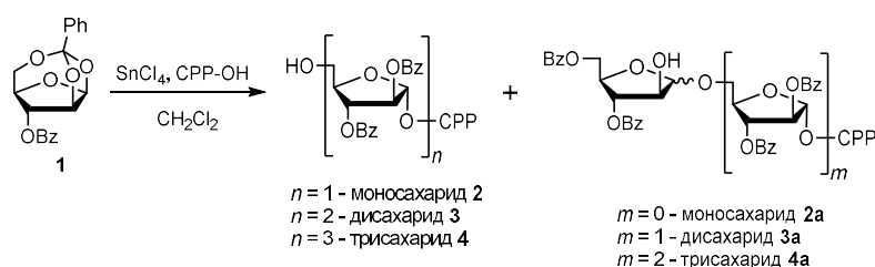
Рис. 1. a – исследуемая реакция олигомеризации ортоэфира 1 , CPP – 4-(3-хлорпропокси)фенил, T = -25 °C или 22 °C. b – схема используемого проточного реактора, M – микромиксер Comet X-01, T – T-образный переходник.
