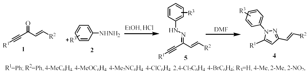
Рисунок 2. Схема синтеза стирилпиразолов
