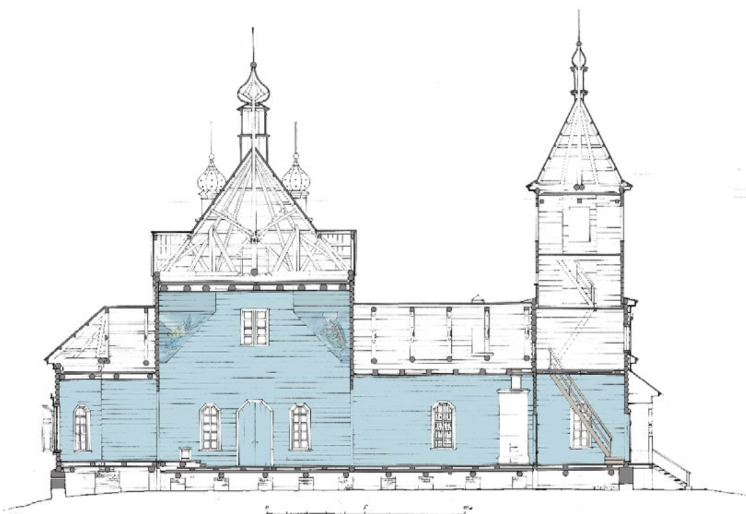
Рис. 4. Реконструкция первоначального облика. Продольный разрез. Рис. А.А. Ермаковой
