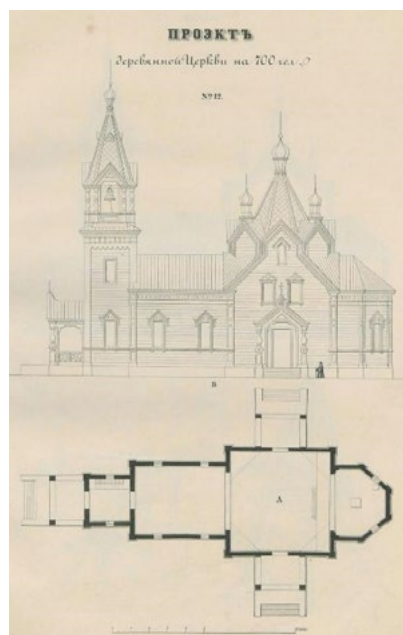
Рис. 1. Образцовый проект 1853 г., по которому была построена церковь Параскевы Пятницы
