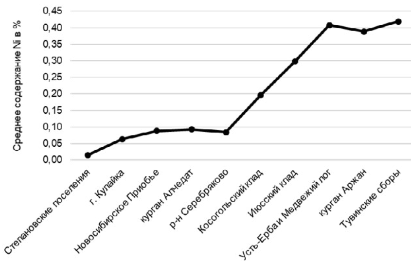
Рис. 2. Средние содержания никеля в изделиях
