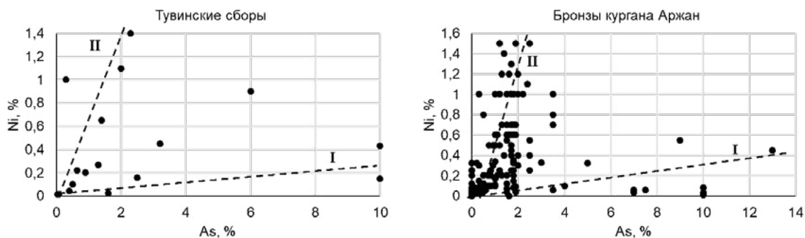
Рис. 4. Корреляция Ni-As в тагарских бронзах Маринской лесостепи
