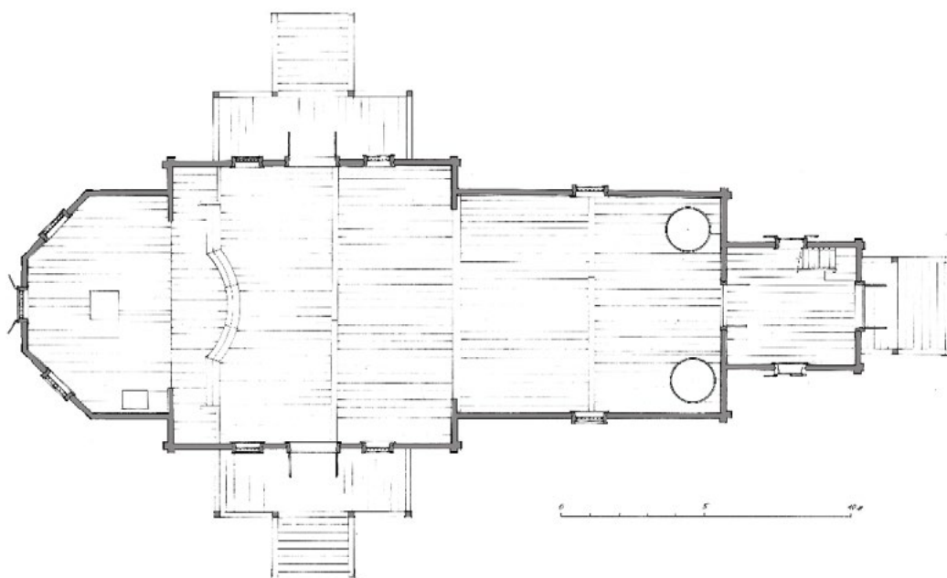
Рис. 3. Реконструкция первоначального облика без обшивки стен. План. Рис. А.А. Ермаковой
