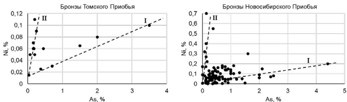
Рис. 3. Корреляция Ni-As в бронзах кулайских изделий
